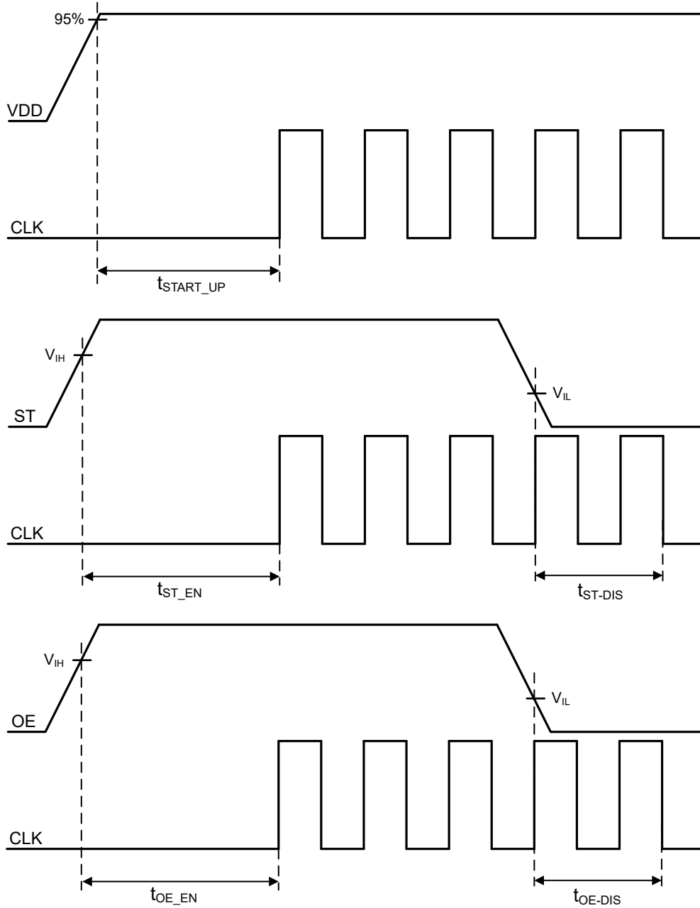
图 6-2. 上电特性
