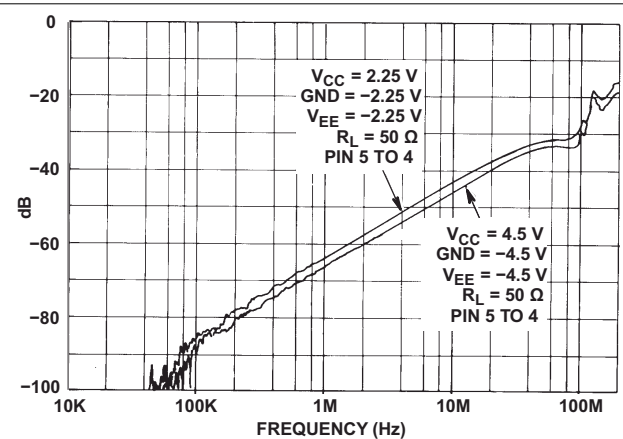
图 5-8. 通道关断带宽 (HC 和 HCT4053)
