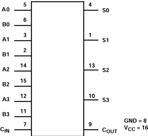
功能方框图
