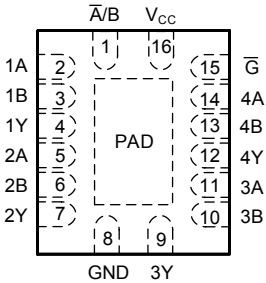
图 4-2. CD74AC157 BQB 封装 ( 顶视图 )
