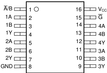
图 4-3. CD74AC157 D 、 N 封装 ( 顶视图 )
