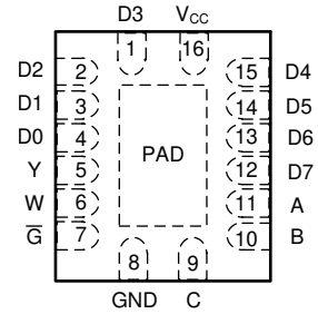
图 3-2. BQB 封装，16 引脚 WQFN ( 透明顶视图 )
