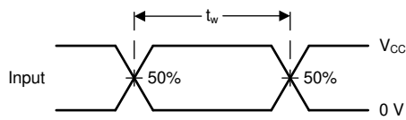
图 6-2. 电压波形，标准 CMOS 输入脉冲持续时间
