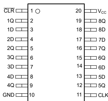
J、DW 或 N 封装 20 引脚 CDIP、PDIP 或 SOIC 顶视图
