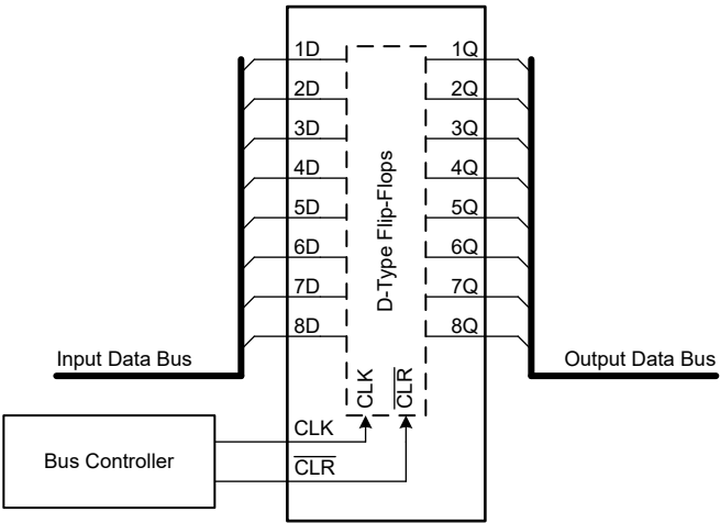
图 8-1. 典型应用图
