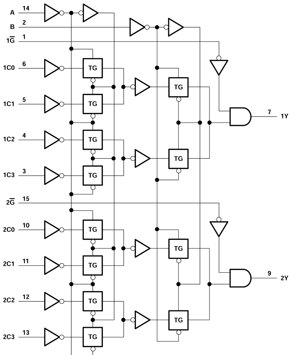
图 6-1. 逻辑图 ( 正逻辑 )
