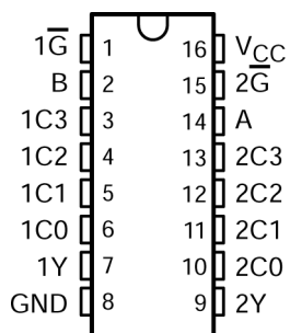
图 3-1. CD54AC153 J 封装，16 引脚 CDIP； CD74AC153 D、N 或 PW 封装；16 引脚 SOIC、PDIP 或 TSSOP（顶视图）
