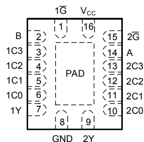
图 3-2. CD74AC153 BQB 封装；16 引脚 WQFN（顶视图）
