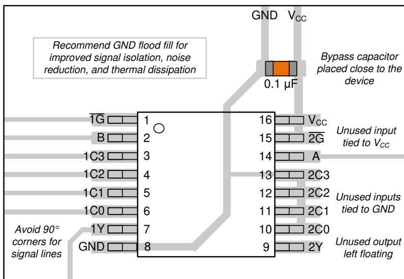
图 7-1. CD74AC153 的示例布局
