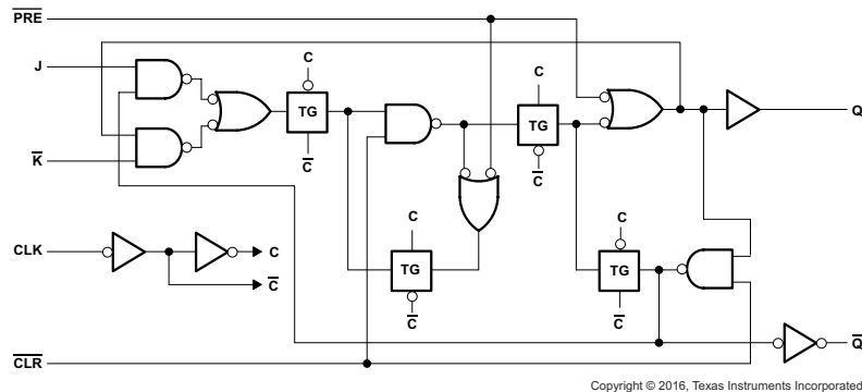
逻辑图
