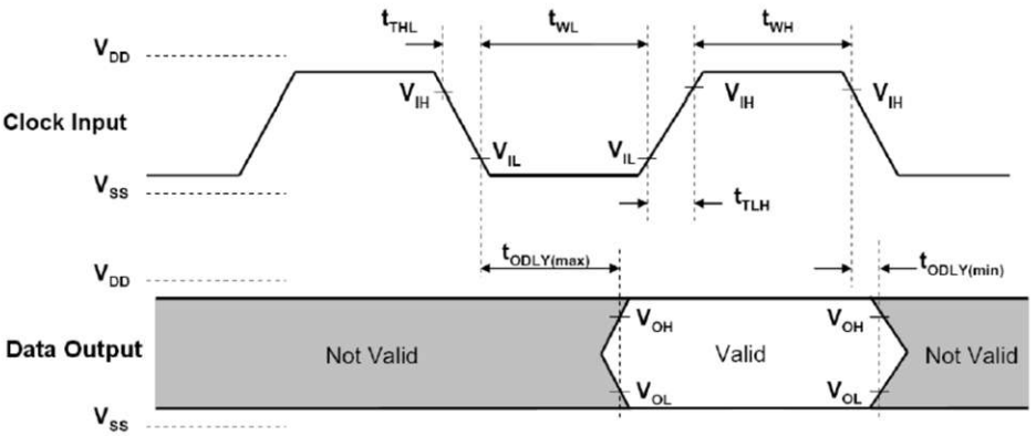
图 6-2. SDIO 默认输出时序
