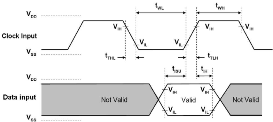
图 6-1. SDIO 默认输入时序
