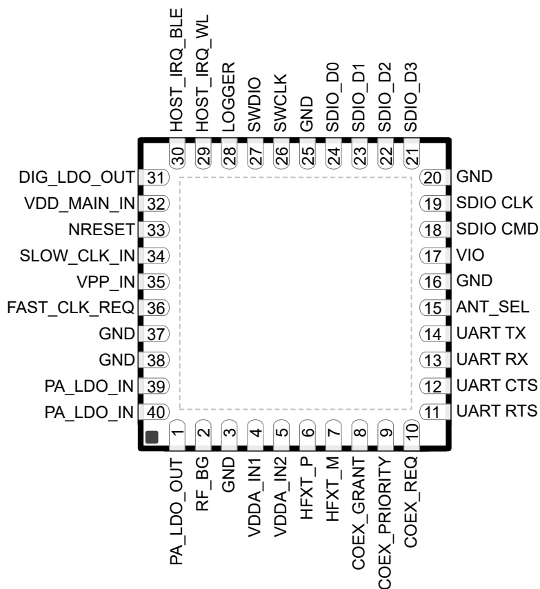
图 5-1. CC3301 引脚图
