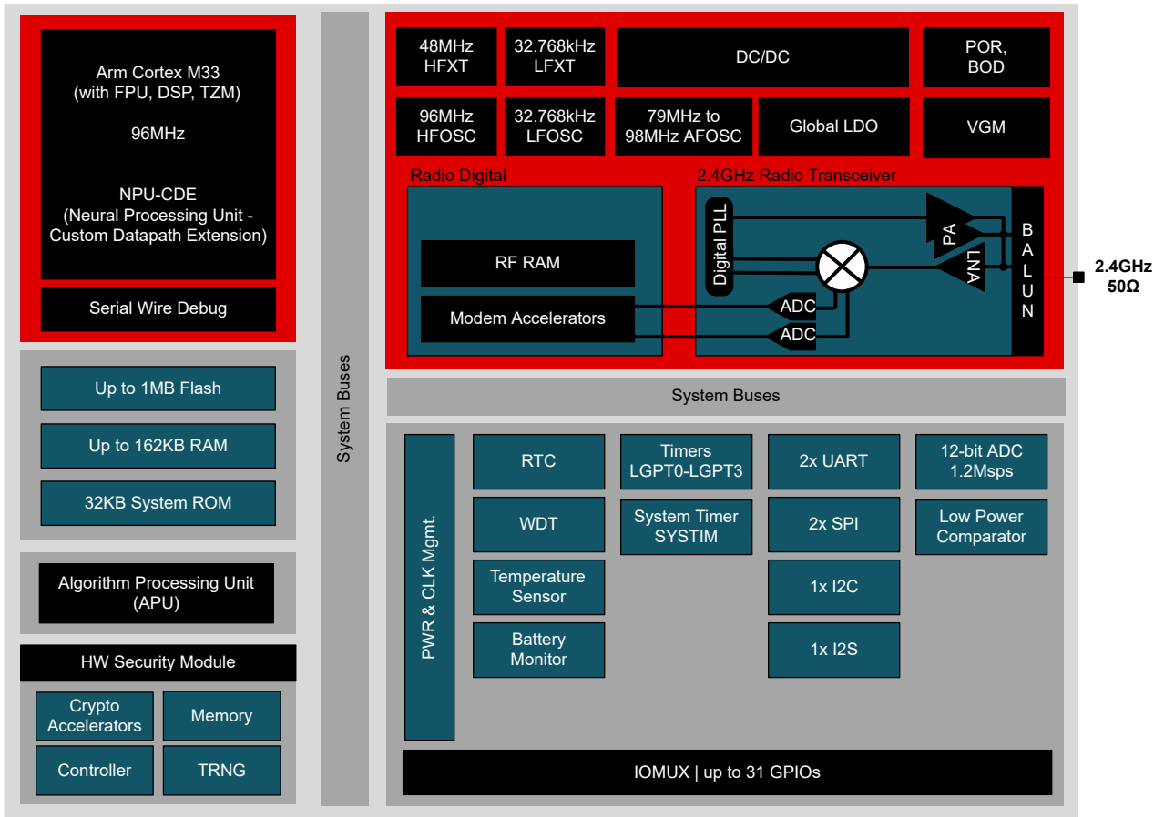
图 4-1. 功能方框图
