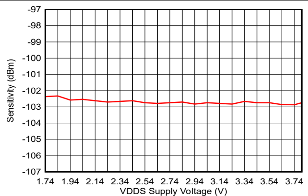
图 7-19. 灵敏度与 VDD 间的关系 (IEEE 802.15.4 PHY)
