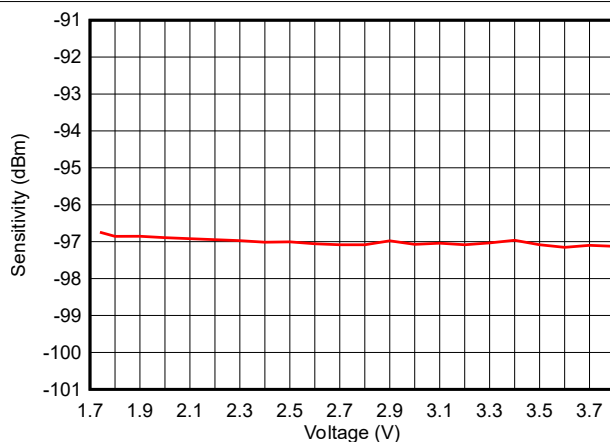
图 7-18. 灵敏度与电源电压 (VDD) 间的关系 (BLE 1Mbps , 2.44GHz )
