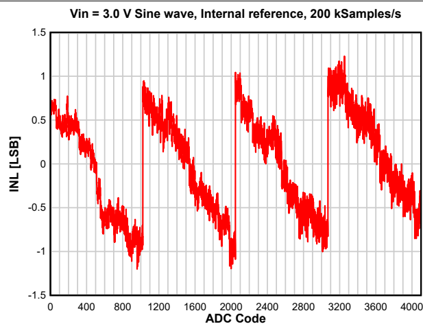
图 8-23. INL versus ADC Code
