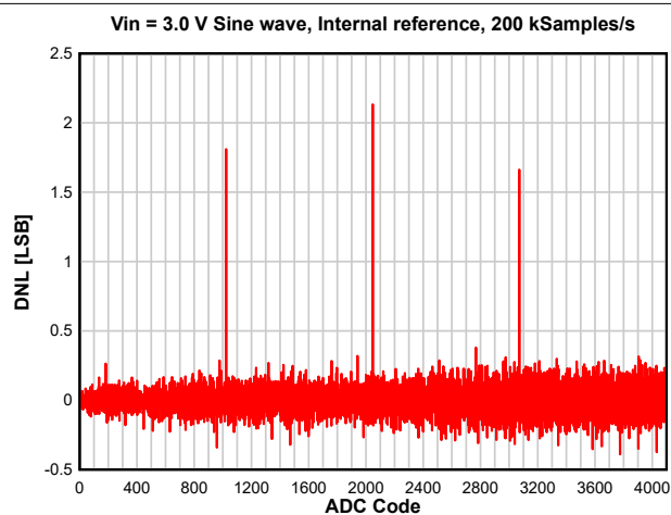
图 8-25. DNL versus ADC Code
