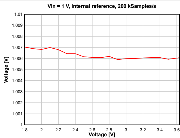
图 8-27. ADC Accuracy versus VDD5
