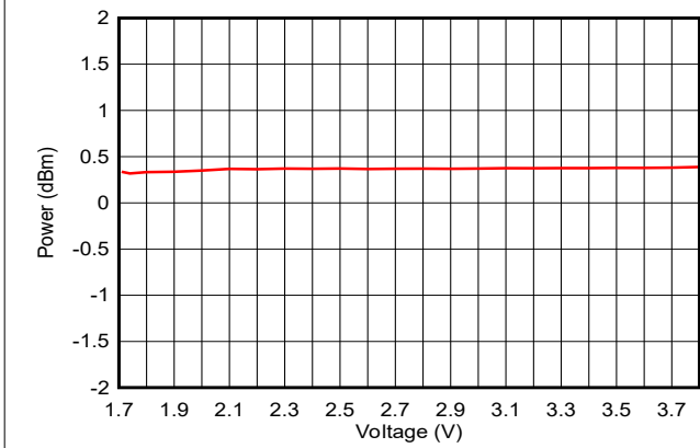
图 7-23. 输出功率与电源电压 (VDD) 间的关系 ( 蓝牙低功耗 1Mbps , 2.44GHz , +0dBm )
