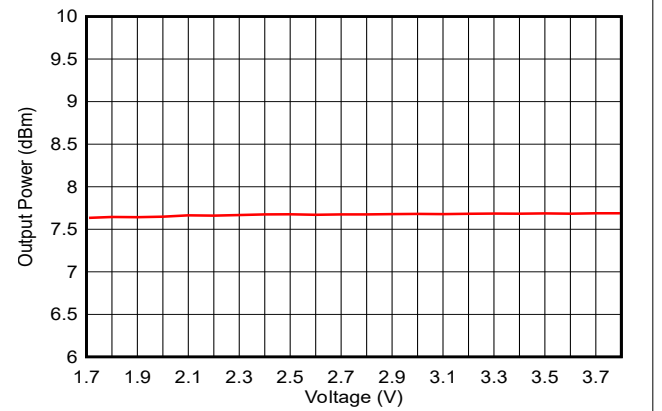
图 7-24. 输出功率与电源电压 (VDD) 间的关系 ( 蓝牙低功耗 1Mbps , 2.44GHz , +8dBm )
