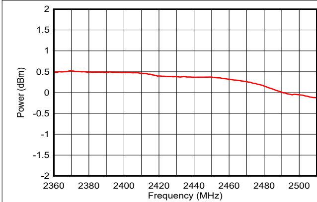
图 7-25. 输出功率与频率间的关系 ( 蓝牙低功耗 1Mbps , 0dBm )
