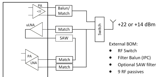
图 8-1. 全性能参考设计方框图
