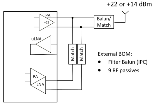
图 8-2. 无开关双 PA 参考设计
