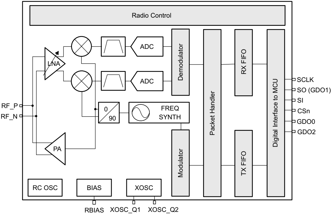
图 1-1. 功能框图
