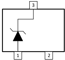
图 5-1. DBZ 封装，3 引脚 SOT-23 (顶视图)
