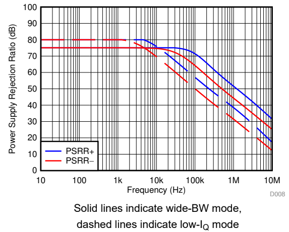
图 6-26. PSRR vs Frequency
