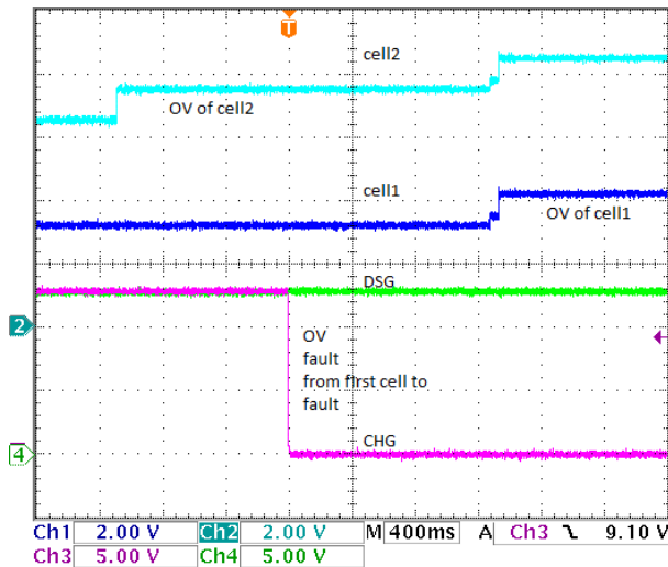
图 10-10. OV Fault Protection
