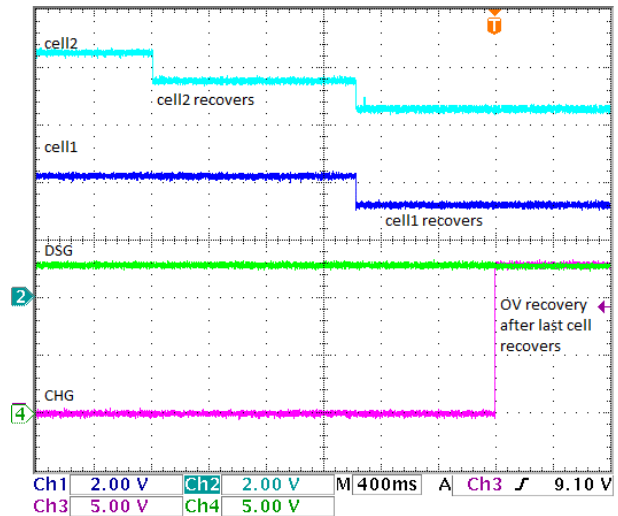
图 10-11. OV Fault Recovery
