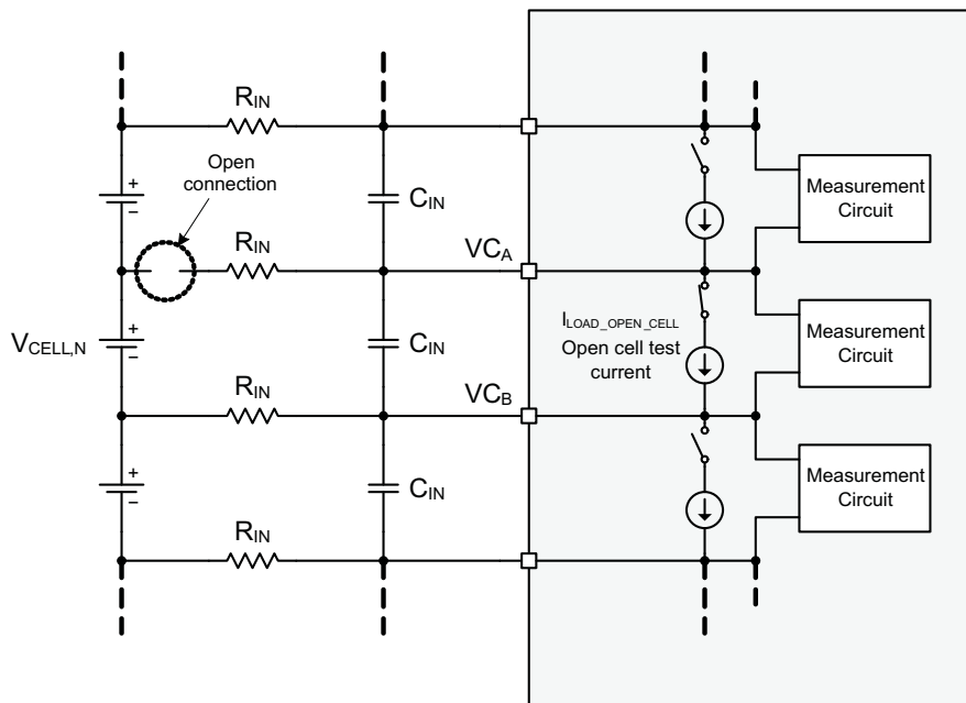
图 9. Open-Cell Check
