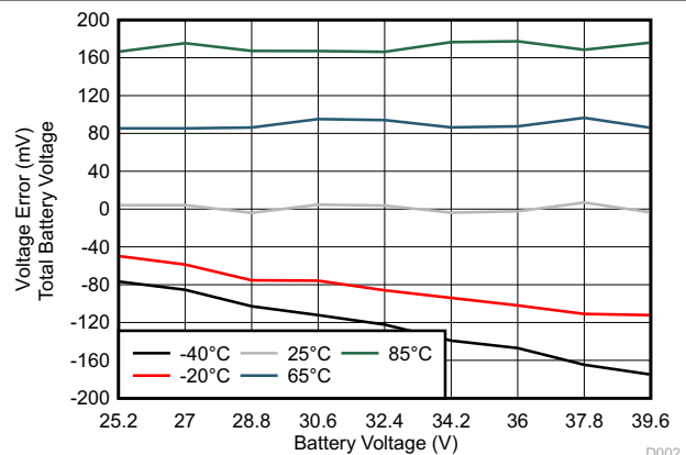
图 8-6. V_{(Err)} Across VIN (0 mA) 9 s
