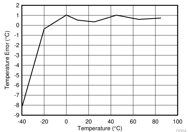
图 8-8. T_{(Err)}
