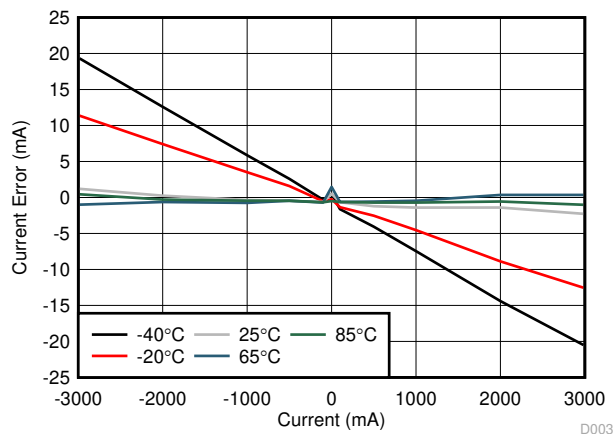
图 8-7. I_{(Err)}
