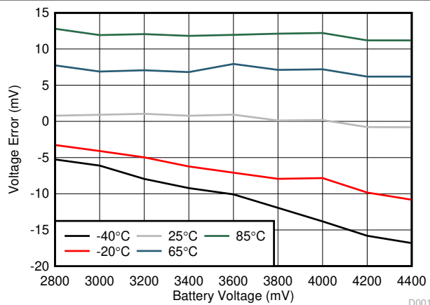
图 8-5. V_{(Err)} Across VIN (0 mA)
