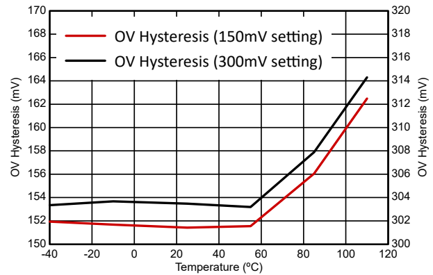
图 6-2. 过压迟滞 ( V_{OVHYS} ) 与温度间的关系
