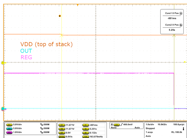
图 8-6. 检测到欠压并禁用稳压器
