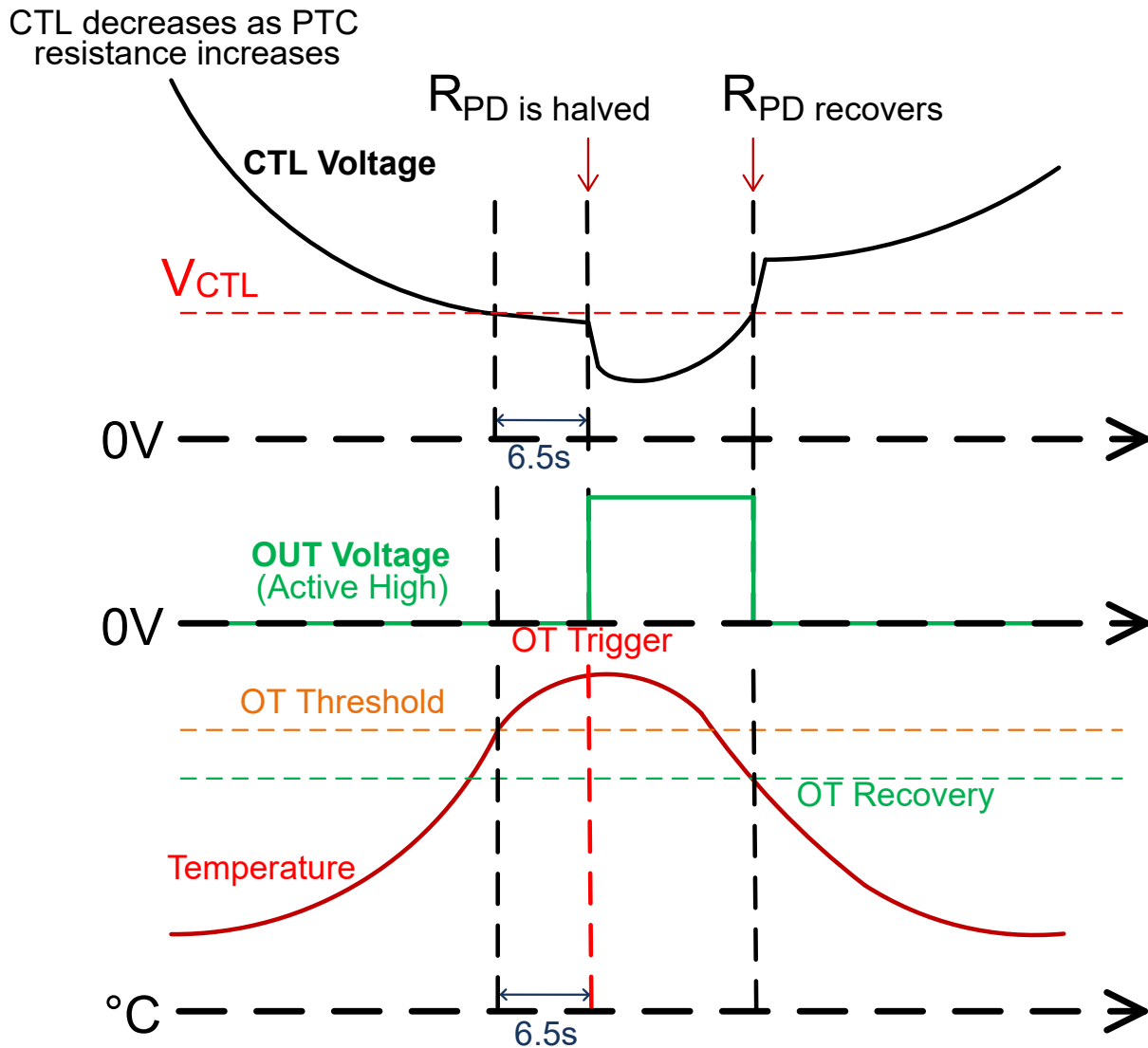
图 8-9. 过热保护
