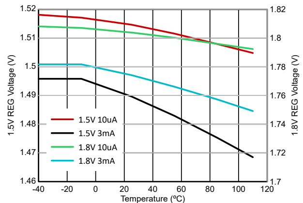
图 6-6. 稳压器输出与温度间的关系 (1.5V 和 1.8V 设置)
