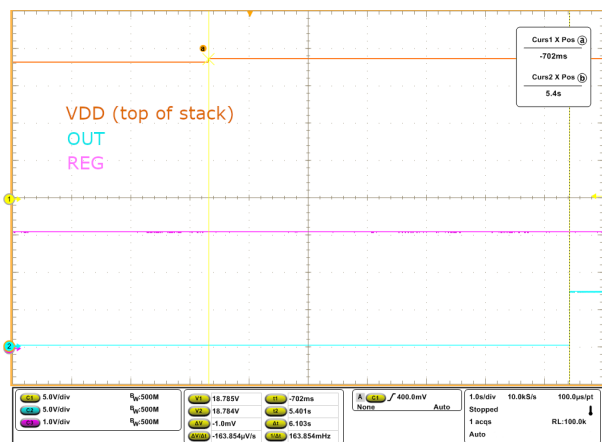
图 8-4. 过压保护触发
