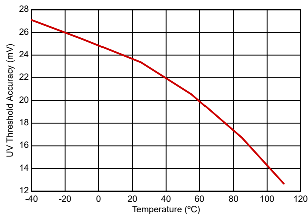
图 6-3. 欠压阈值精度与温度间的关系
