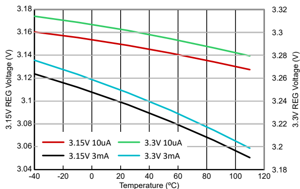
图 6-8. 稳压器输出与温度间的关系 (3.15V 和 3.3V 设置)
