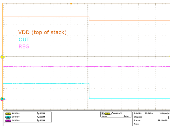
图 8-5. 过压保护恢复
