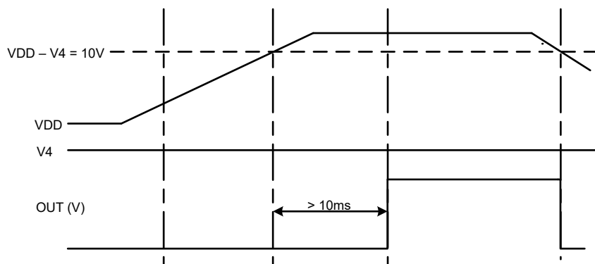
图 7-4. 客户测试模式的时序
