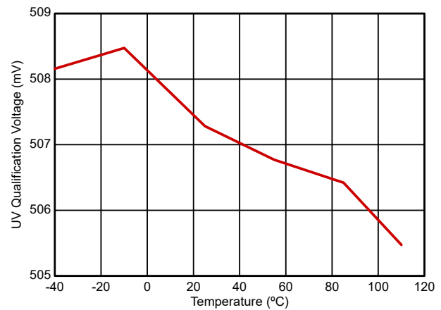
图 6-4. 欠压鉴定电压 ( V_{UVQUAL} ) 与温度间的关系
