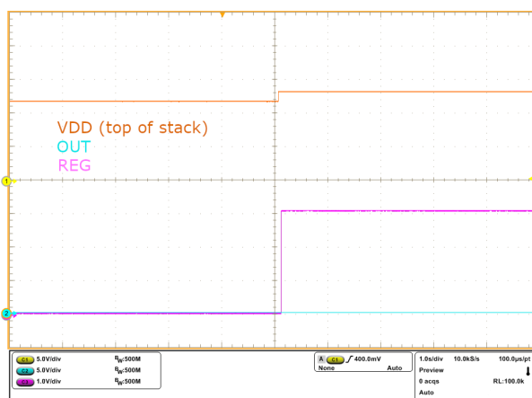
图 8-7. 从欠压恢复并重新启用稳压器
