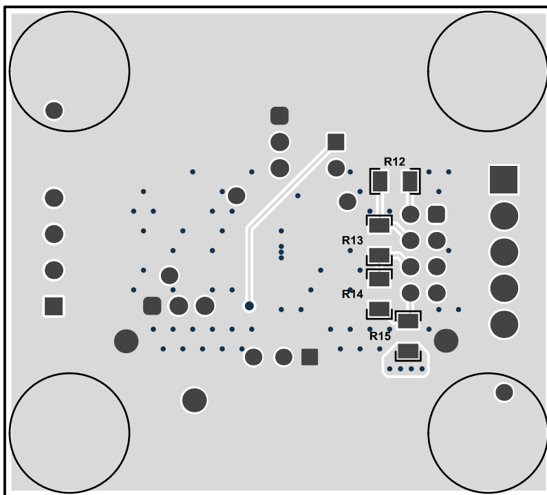
图 8-12. BQ2969T 两层电路板布局布线 - 底层
