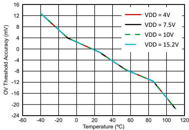
图 6-1. 过压阈值精度 ( V_{OA} ) 与温度间的关系
