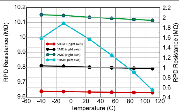
图 6-12. CTL 下拉电阻 ( R_{PD} ) 与温度间的关系
