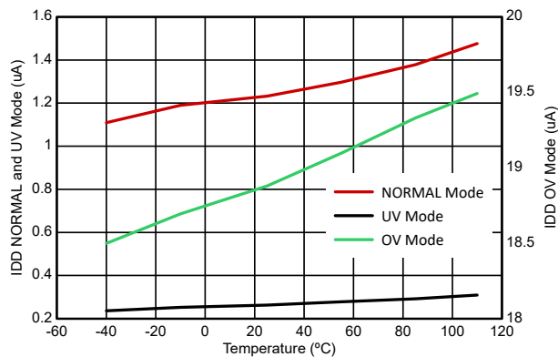
图 6-5. I_{DD} 与温度间的关系
