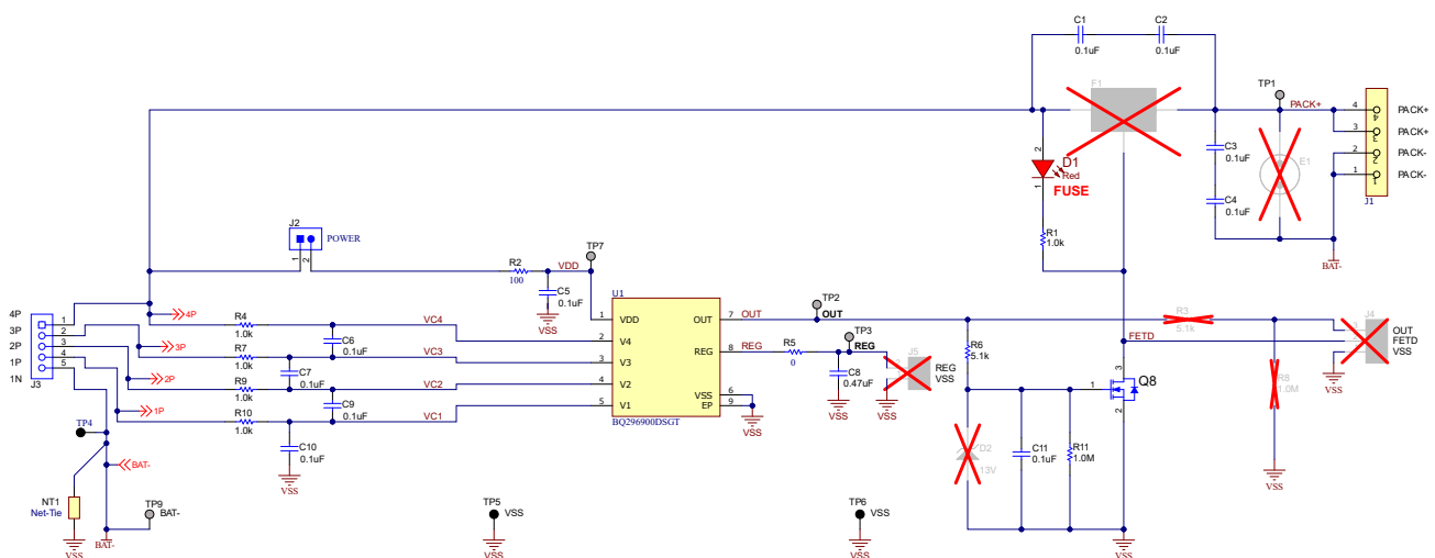
图 8-2. BQ2969 4 节串联电芯原理图 - 保护器和保险丝熔断电路
