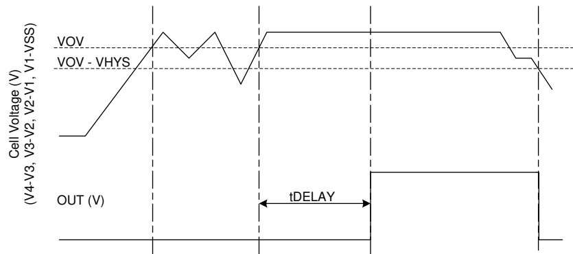
图 7-1. OUT 过压检测时序
