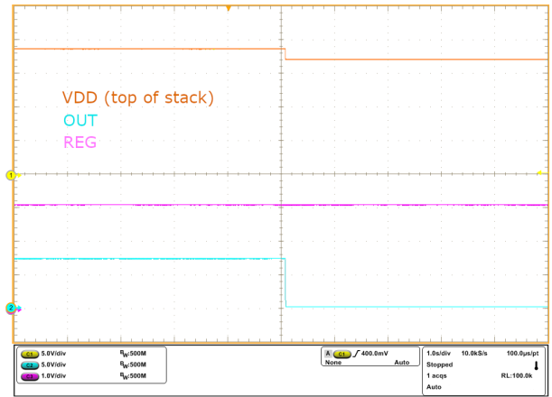
图 8-5. 过压保护恢复
