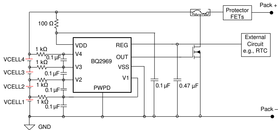
图 8-1. BQ2969 4 节串联电芯典型实现方式 (简化原理图)
