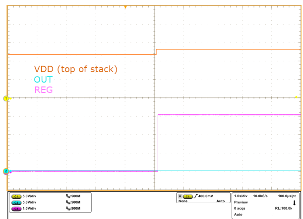
图 8-7. 从欠压恢复并重新启用稳压器
