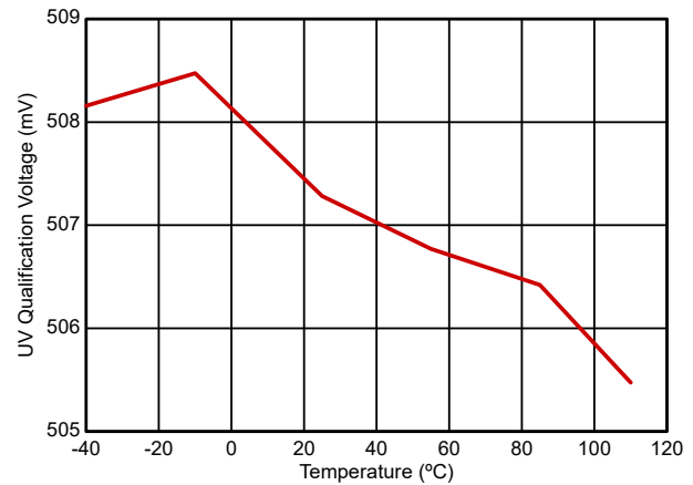
图 6-4. 欠压鉴定电压与温度间的关系
