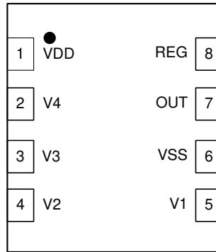
图 5-1. 2 节至 4 节串联 BQ2969 DSG 封装、8 引脚 WSON (顶视图)
