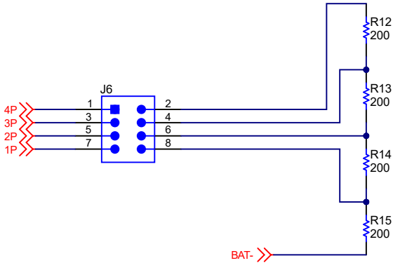
图 8-3. BQ2969 4 节串联电芯原理图 - 电芯模拟器电路
