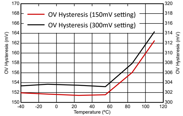
图 6-2. 过压迟滞与温度间的关系
