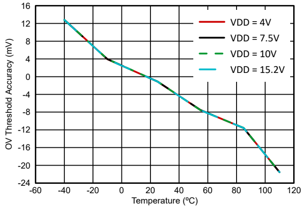
图 6-1. 过压阈值精度与温度间的关系
