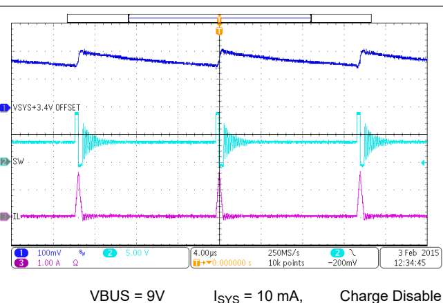
图 9-9. PFM Switching Waveform
