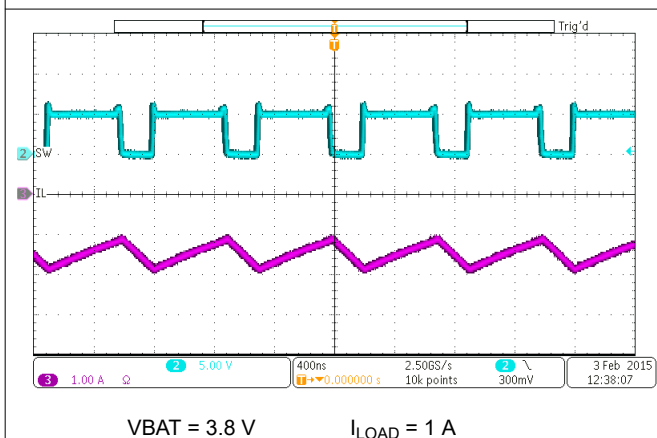
图 9-10. Boost Mode Switching Waveform
