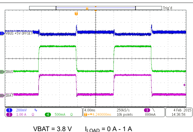
图 9-11. Boost Mode Load Transient
