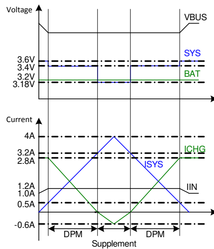
图 8-3. DPM Response
