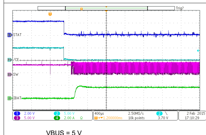
图 9-4. Charge Enable
