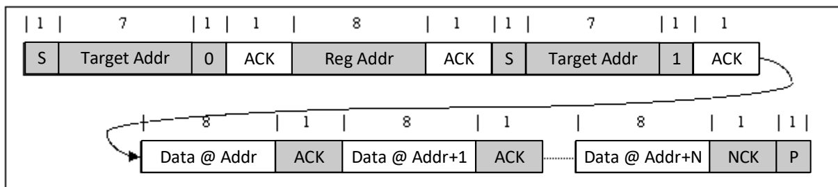
图 8-16. Multi-Read
