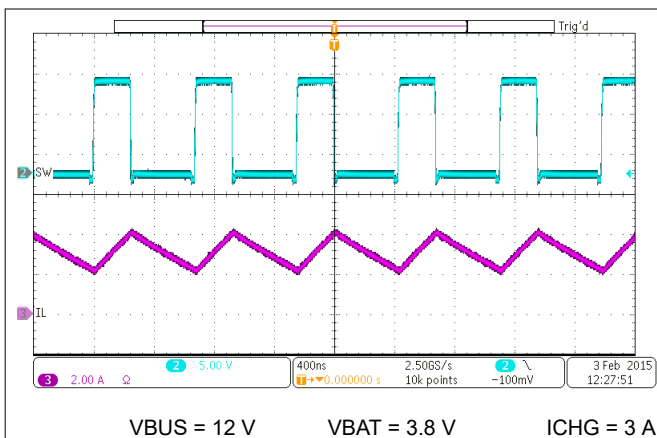
图 9-8. PWM Switching Waveform
