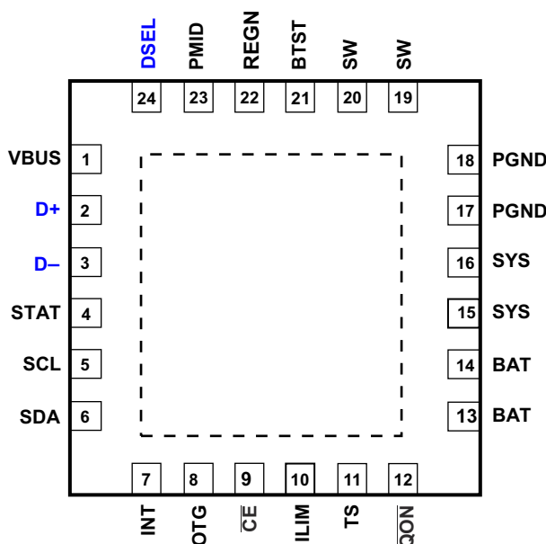
图 6-1. BQ25895M RTW (WQFN) Top View
