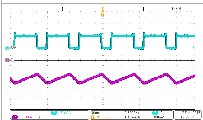
图 9-10. PWM Switching Waveform
