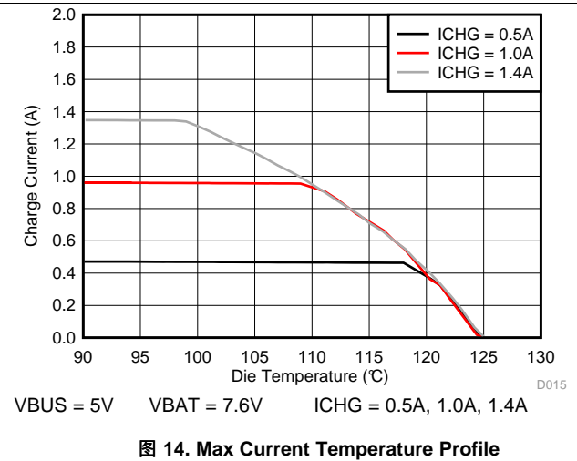
图 14. Max Current Temperature Profile
