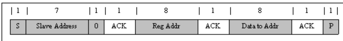
图 30. Single Write
