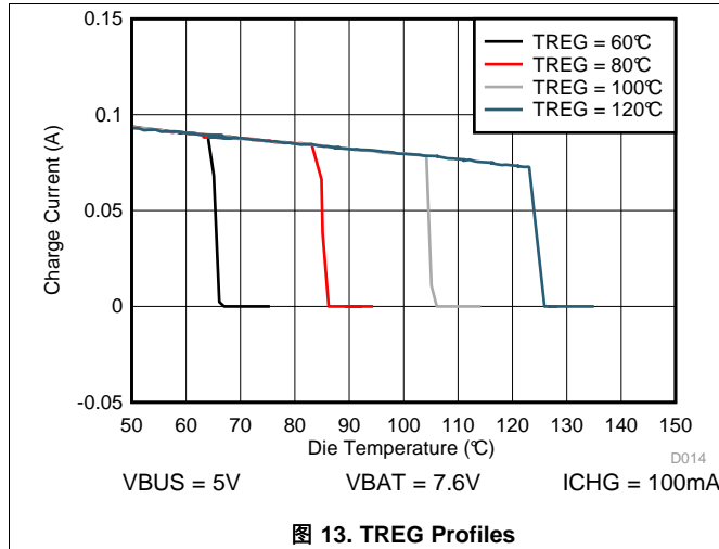
图 13. TREG Profiles
