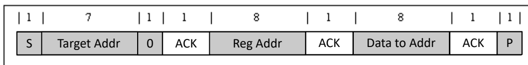
图 8-11. 单独写入
