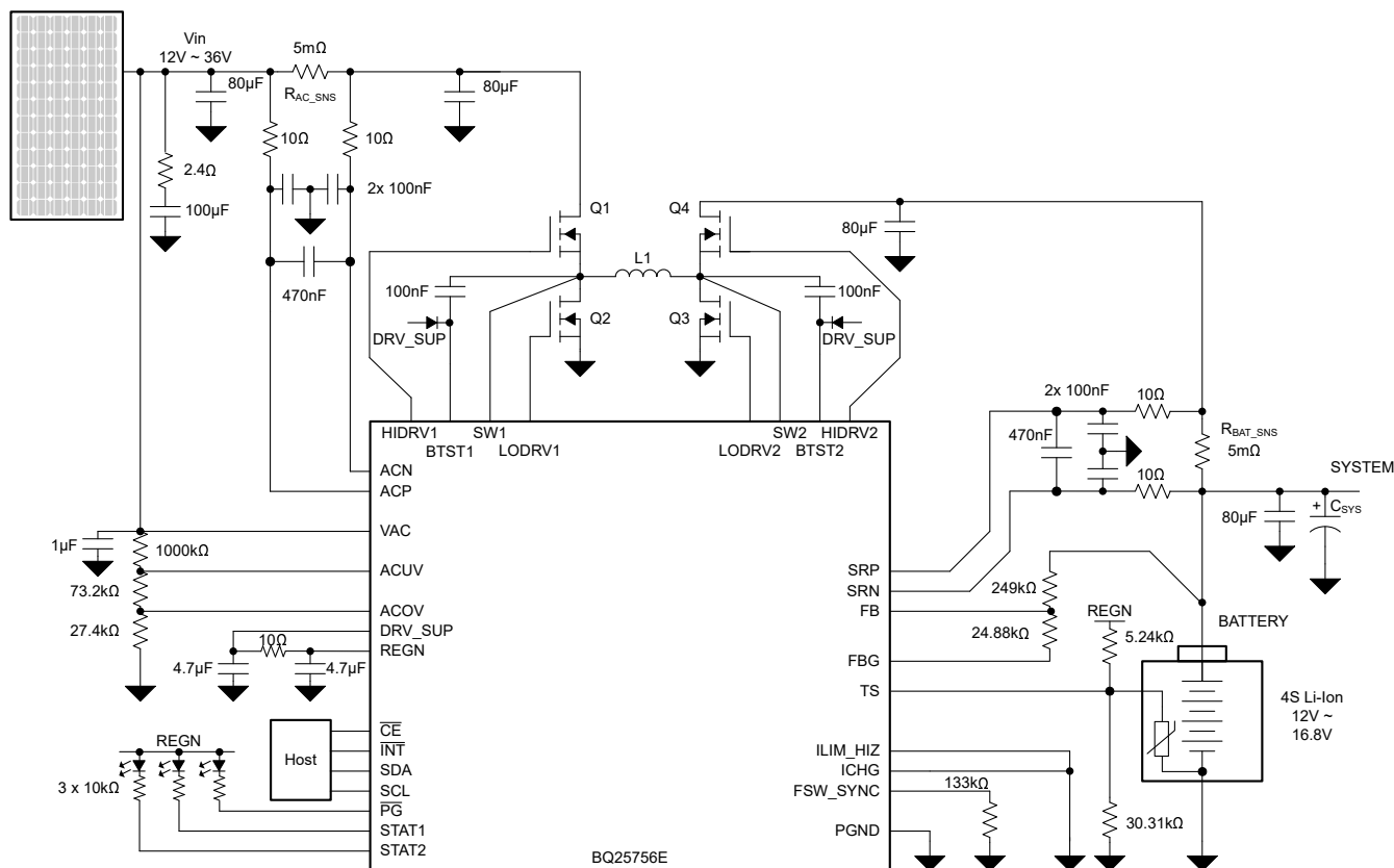
图 9-1. BQ25756E：采用自主 MPPT 算法的太阳能充电，以最大 15A 充电电流为 4 节串联电池充电
