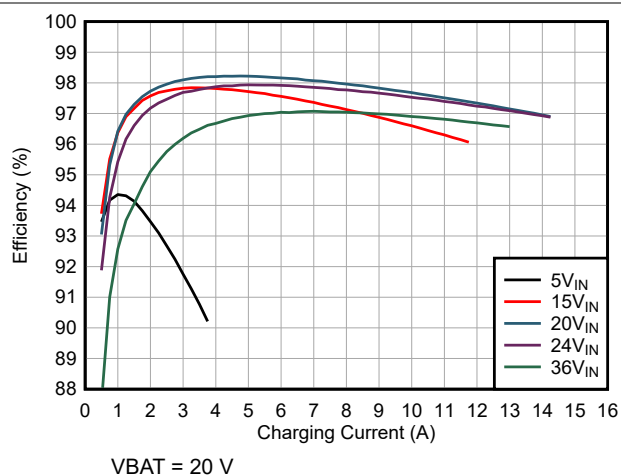
图 7-2. 充电效率与充电电流间的关系 (5 节串联电池配置)
