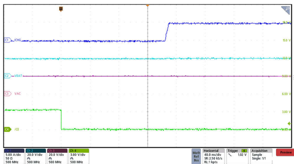
图 9-5. 5A ICHG 下通过 I 2 C 实现的充电启用
