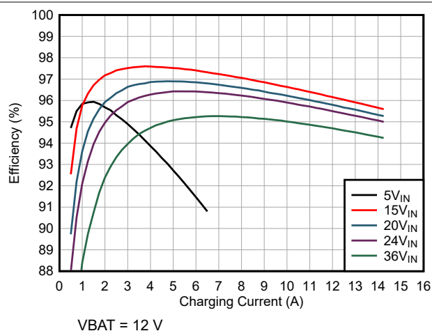
图 7-1. 充电效率与充电电流间的关系 (3 节串联电池配置)
