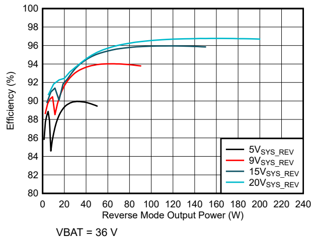
图 7-11. 反向模式效率 (9 节串联电池配置)
