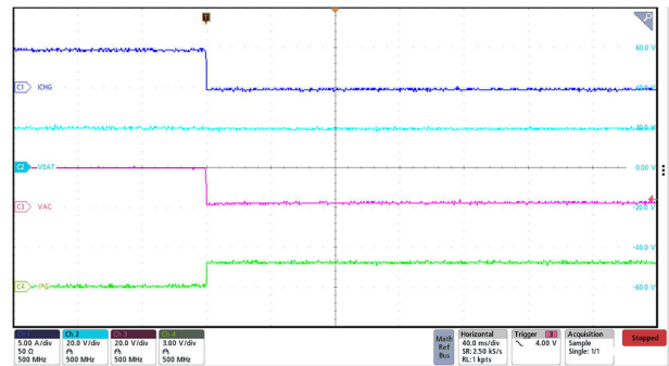
图 9-4. 5A ICHG 下的 VAC 拔下断电
