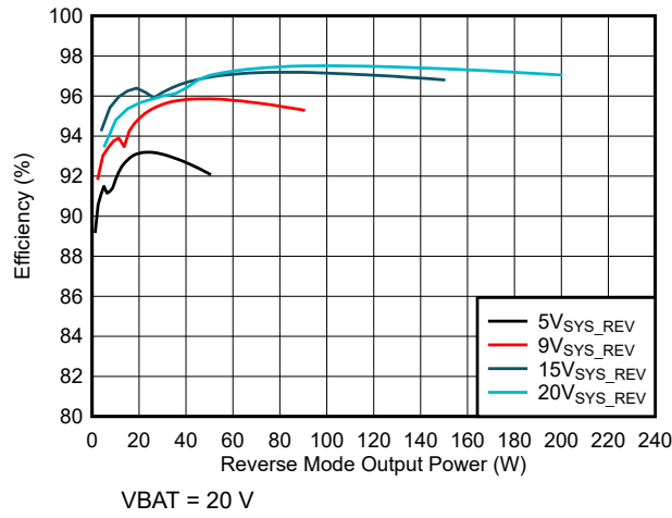
图 7-9. 反向模式效率 (5 节串联电池配置)
