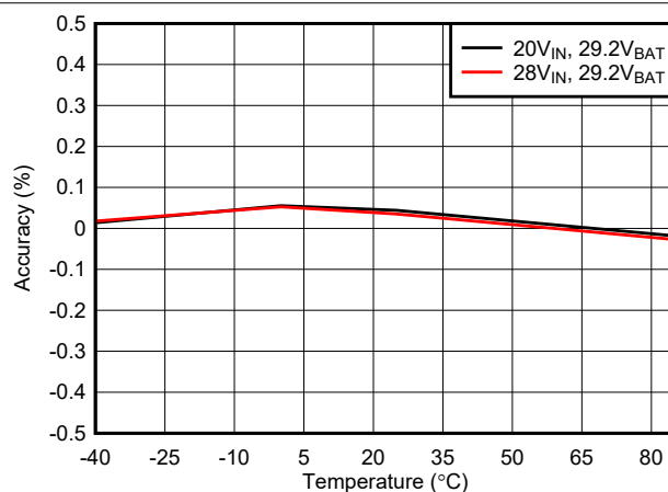
图 7-4. 充电电压精度与温度间的关系
