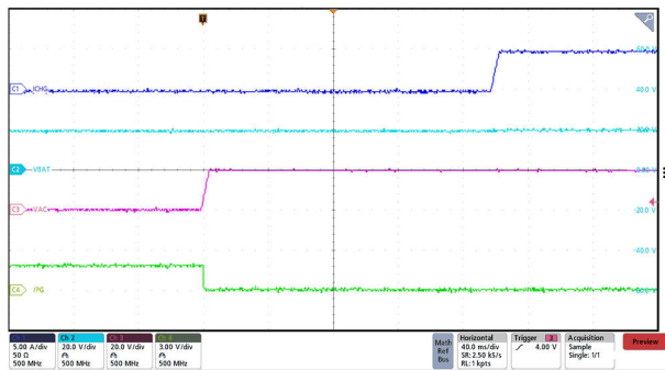
图 9-3. 5A ICHG 下的 VAC 插入上电
