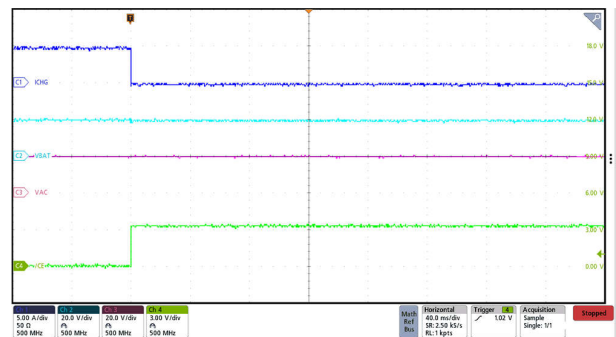
图 9-8. 5A ICHG 下通过 CE 引脚实现的充电禁用
