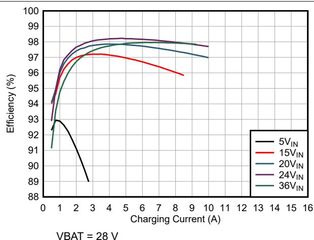
图 7-3. 充电效率与充电电流间的关系 (7 节串联电池配置)
