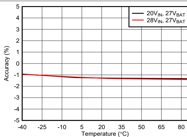
图 7-5. 充电电流精度与温度间的关系
