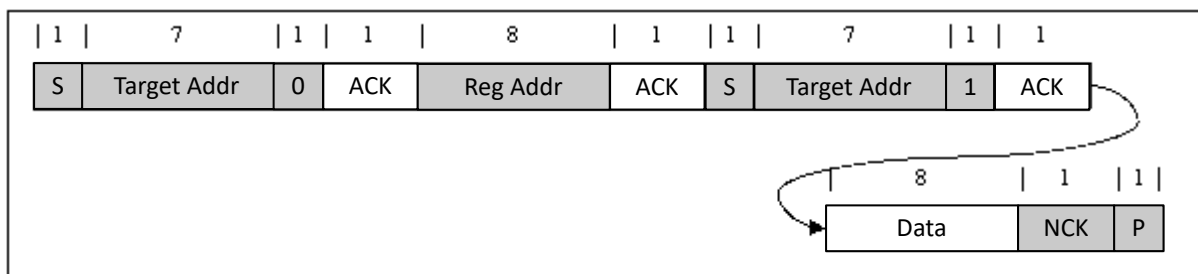
图 8-12. 单次读取
