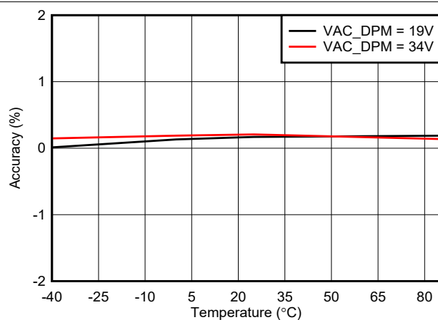
图 7-7. 输入电压 (VAC_DPM) 调节精度与温度间的关系
