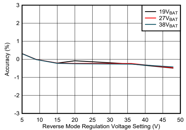
图 5-12. 反向模式输出电压精度与 VAC_REV 设置间的关系
