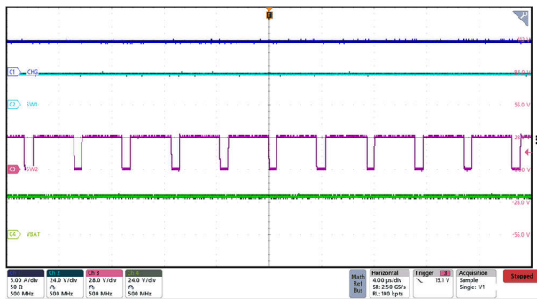
图 7-10. 升压开关波形
