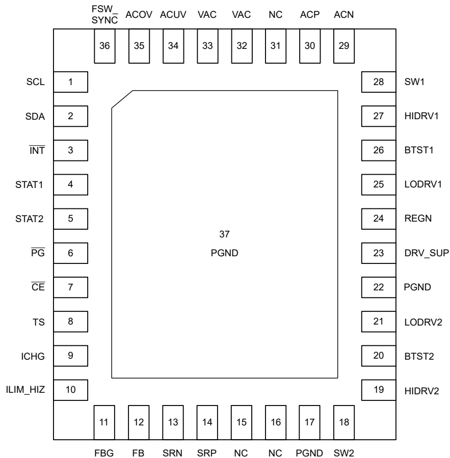
图 4-1. BQ25756 , RRV 封装 36 引脚 VQFN 顶视图
