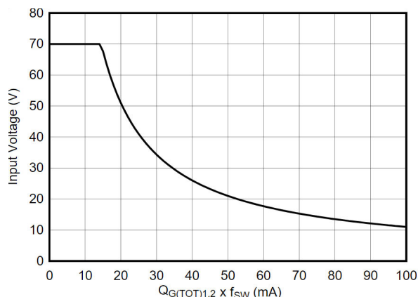
图 6-2. REGN LDO 安全工作区 (SOA)
