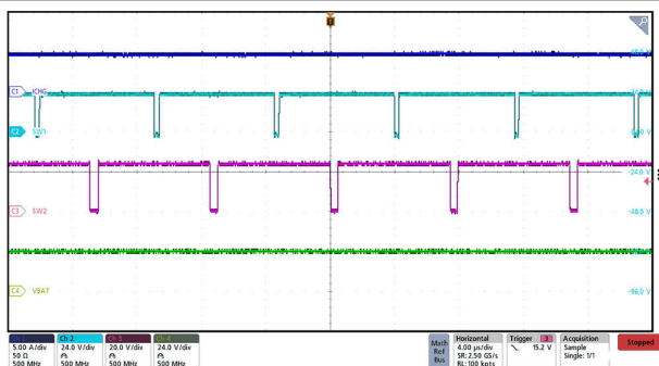
图 7-9. 降压开关波形
