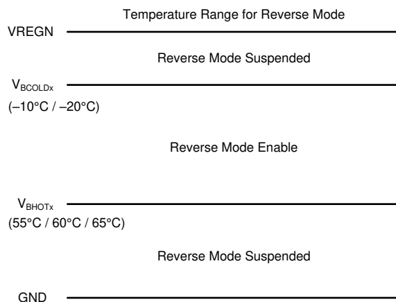
图 6-5. 反向模式下的 TS 引脚热敏电阻检测阈值
