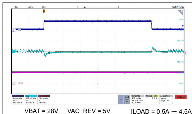
图 7-15. 反向模式降压瞬态响应
