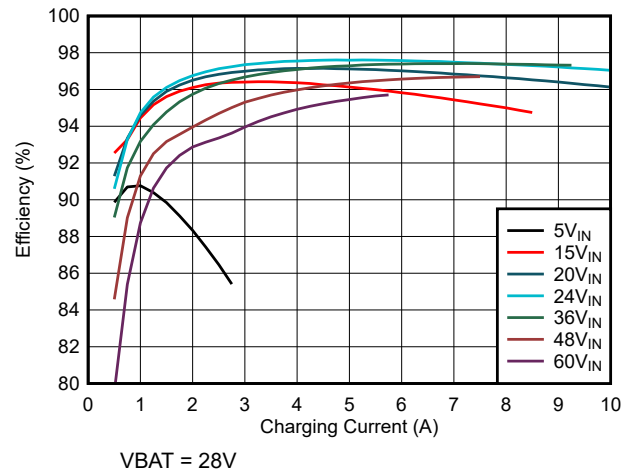
图 5-2. 充电效率与充电电流间的关系 (7 节串联电池配置)
