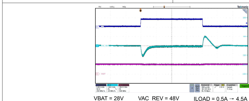
图 7-17. 反向模式升压瞬态响应
