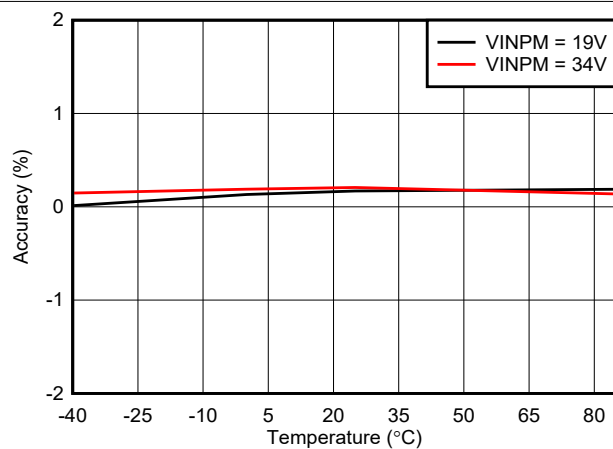
图 5-5. 充电电流精度与温度间的关系
