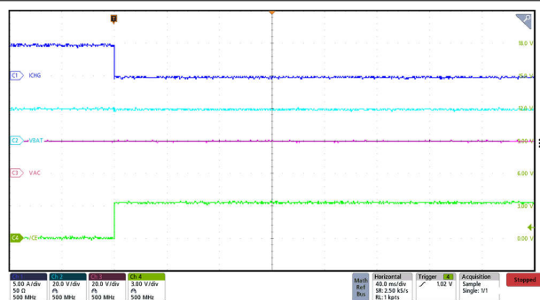
图 7-8. 5A ICHG 下通过 CE 引脚实现的充电禁用
