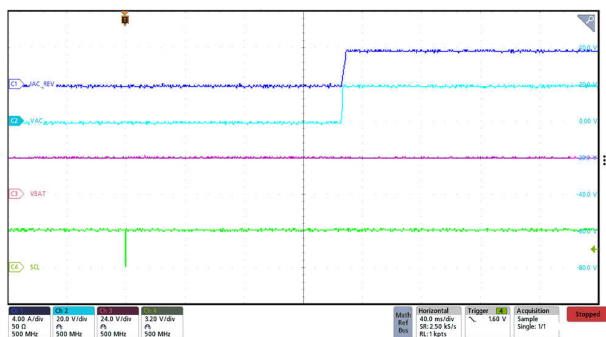
图 7-13. 4A 负载下的反向模式上电
