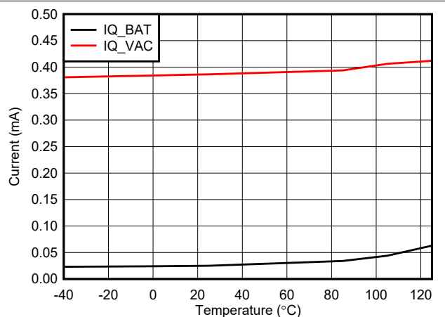
图 5-6. VBAT = 28V 时电池和输入静态电流与温度间的关系
