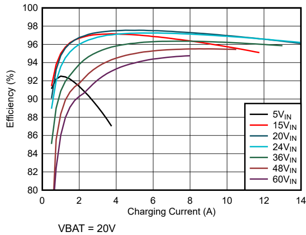
图 5-1. 充电效率与充电电流间的关系 (5 节串联电池配置)
