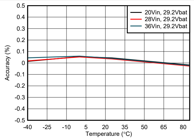
图 5-4. 充电电压精度与温度间的关系
