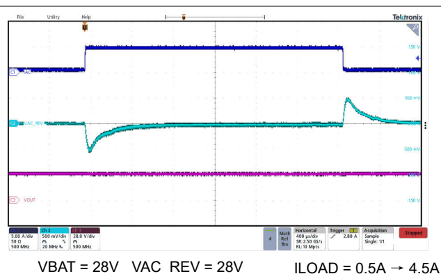
图 7-16. 反向模式降压/升压瞬态响应
