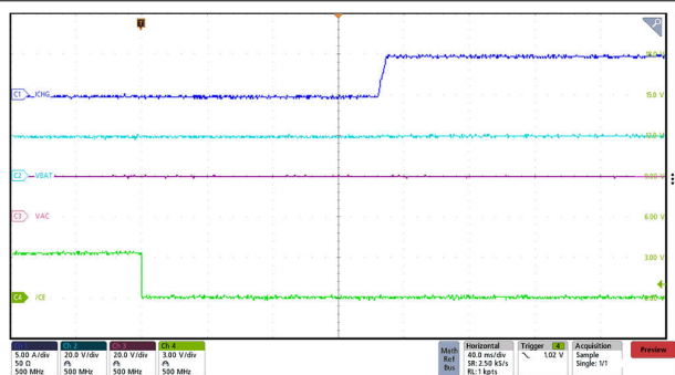
图 7-5. 5A ICHG 下通过 I 2 C 实现的充电启用
