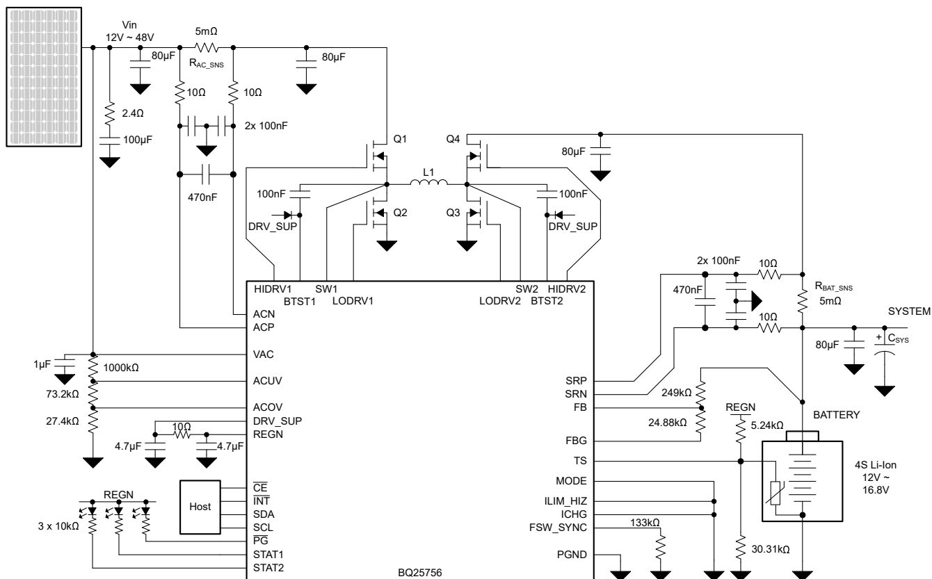
图 7-1. BQ25756：采用自主 MPPT 算法的太阳能充电，以最大 15A 充电电流为 4 节串联电池充电
