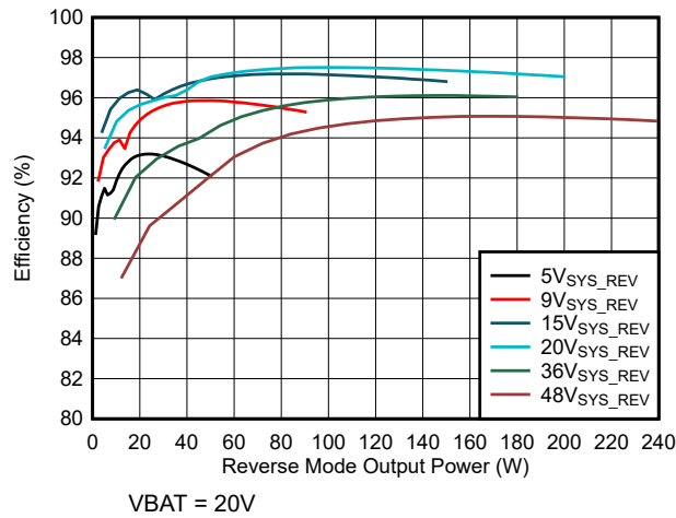
图 5-9. 反向模式效率 (5 节串联电池配置)
