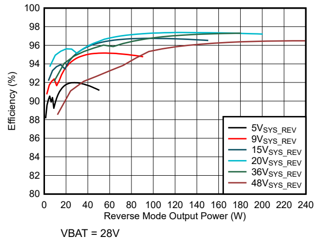
图 5-10. 反向模式效率 (7 节串联电池配置)
