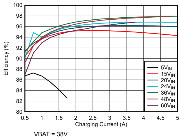
图 5-3. 充电效率与充电电流间的关系 (10 节串联电池配置)
