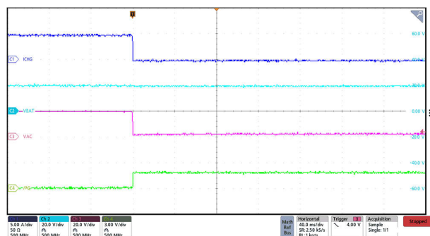
图 7-4. 5A ICHG 下的 VAC 拔下断电
