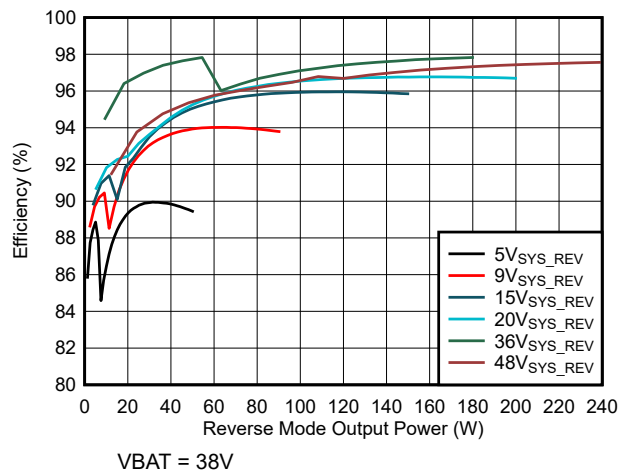
图 5-11. 反向模式效率 (10 节串联电池配置)
