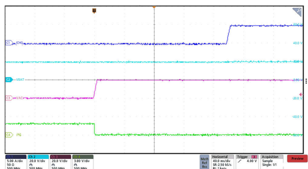
图 7-3. 5A ICHG 下的 VAC 插入上电
