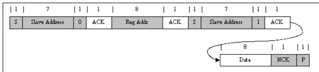
图 9-9. 单次读取
