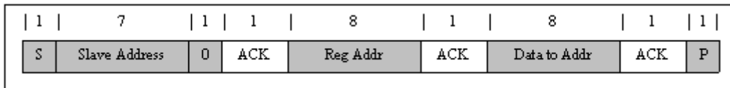
图 9-8. 单独写入
