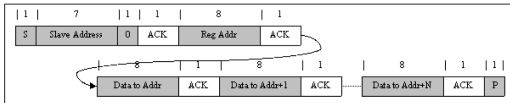
图 9-10. 多重写入
