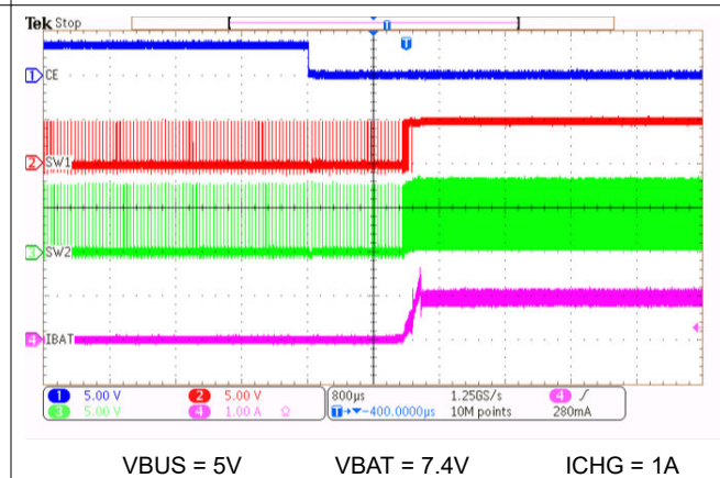
图 8-5. 通过 \overline{CE} 引脚启用充电
