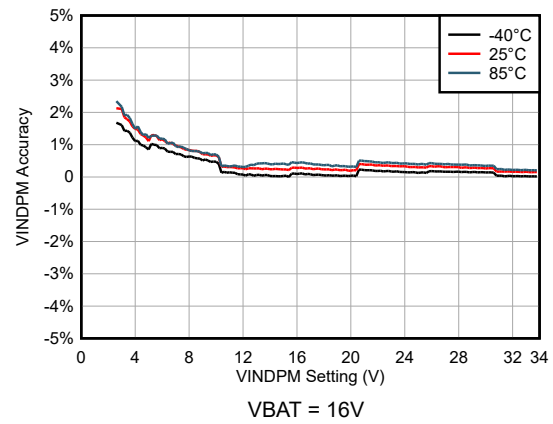
图 5-14. VINDPM 精度
