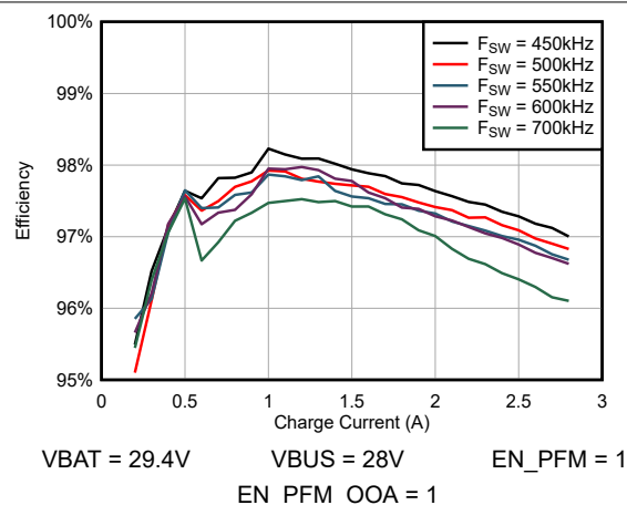
图 5-8. 不同开关频率下 7 节充电效率与充电电流间的关系
