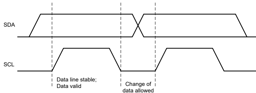
图 6-12. I 2 C 总线上的位传输
