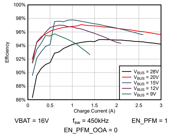
图 5-2. 4 节 充电效率与充电电流间的关系
