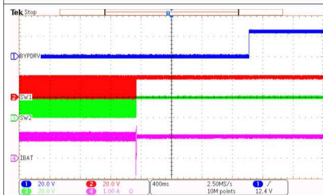
图 8-8. 电池插入检测
