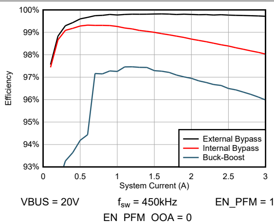
图 5-7. 旁路模式效率与系统电流间的关系
