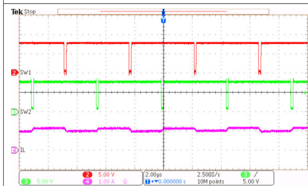
图 8-10. 降压/升压从内部旁路至外部旁路的转换
