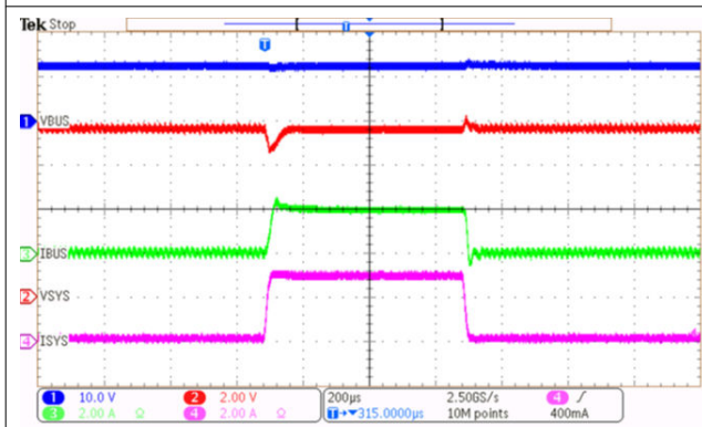
图 8-14. 具有 OOA 的正向升压模式 PFM
