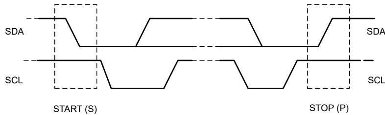
图 6-13. I 2 C 总线上的 START 和 STOP 条件
