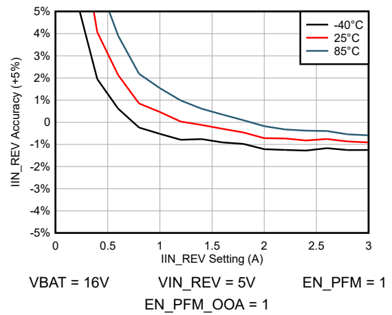
图 5-16. IIN_REV 精度
