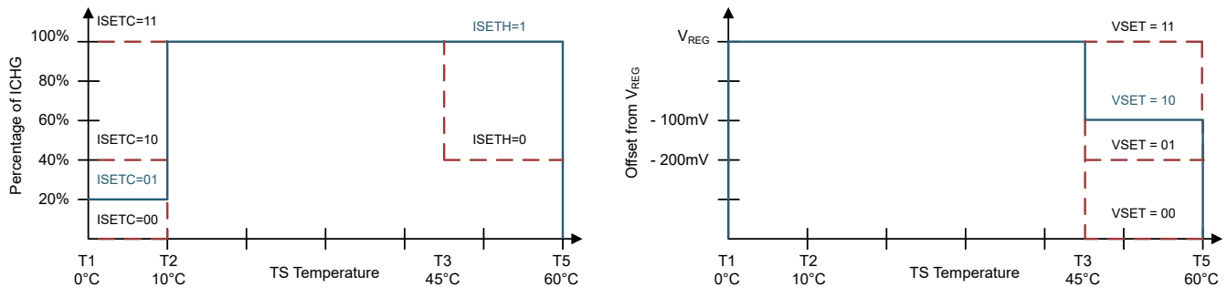
图 6-4. TS 充电值
