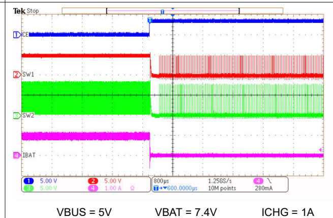
图 8-7. 通过 \overline{CE} 引脚禁用充电
