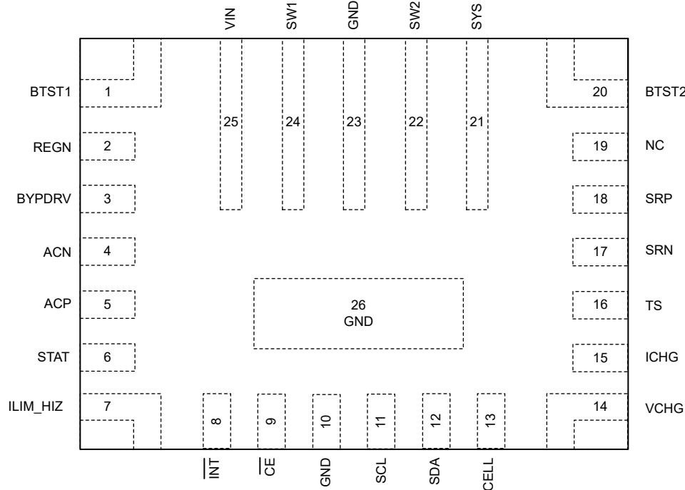
图 4-1. BQ25692-Q1 RBA 封装 26 引脚 WQFN-HR (带可湿性侧面) 顶视图
