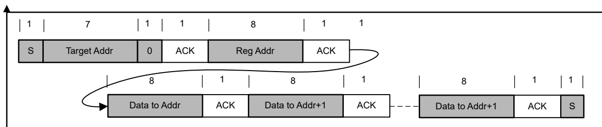
图 6-18. 多重写入
