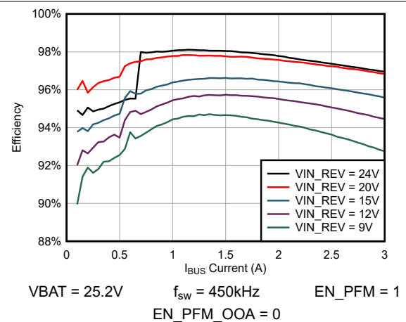
图 5-6. 6 节 电池 OTG 效率与 OTG 电流间的关系
