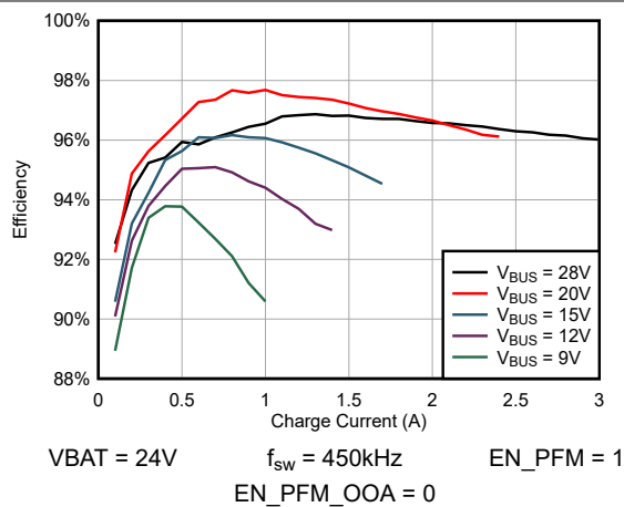
图 5-3. 6 节 充电效率与充电电流间的关系
