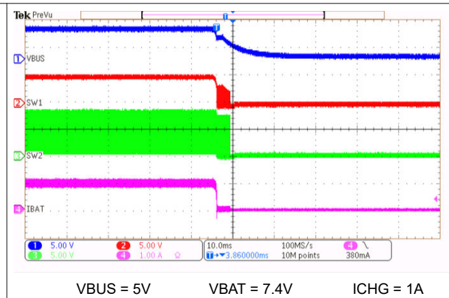
图 8-3. 启用充电时的适配器拔出
