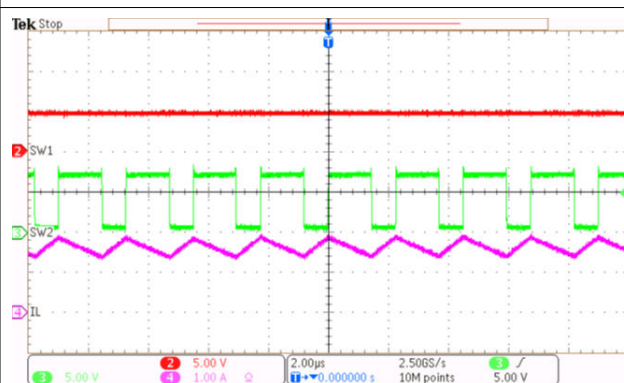
图 8-11. 正向降压模式 CCM
