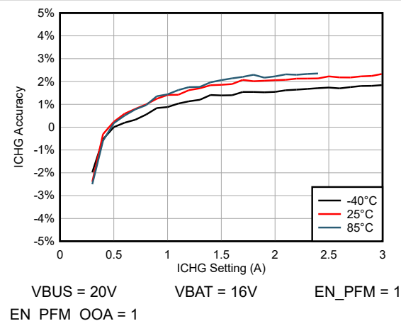
图 5-12. 充电电流精度
