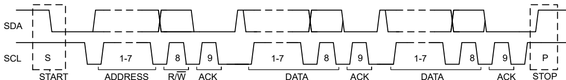
图 6-15. I 2 C 总线上的完整数据传输
