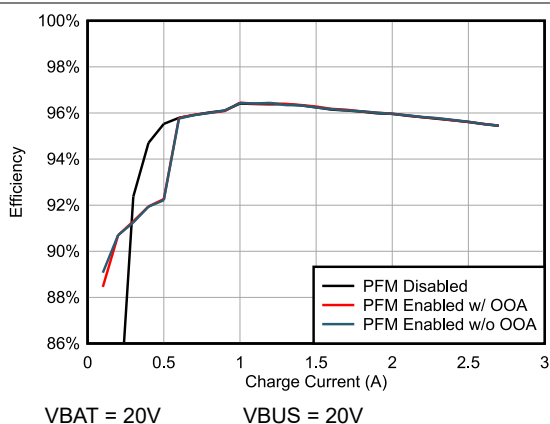
图 5-9. 不同 PWM/PFM/OOA 模式下 5 节充电效率与充电电流间的关系
