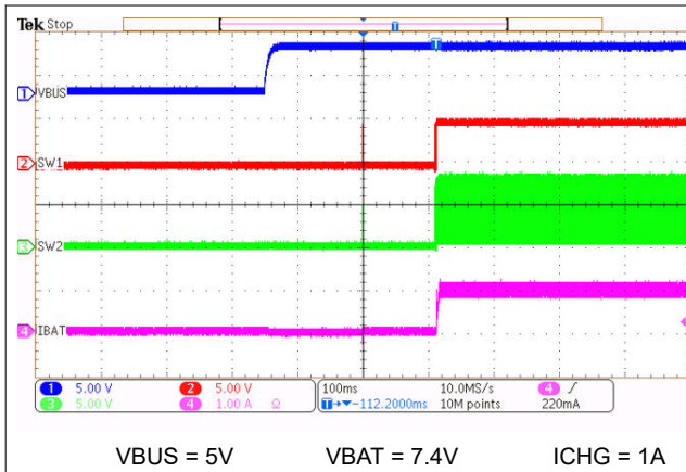
图 8-2. 启用充电时的适配器插入
