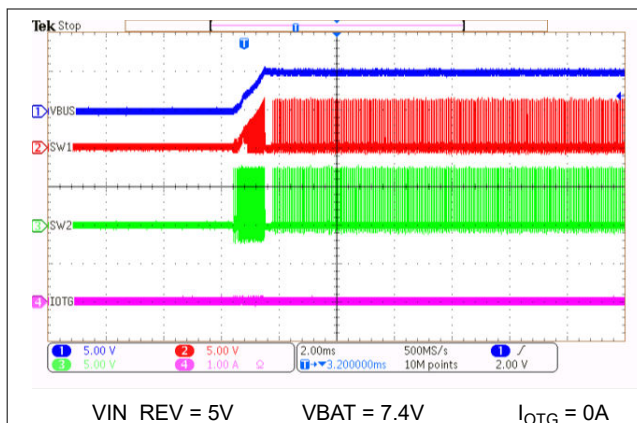
图 8-20. 在无 OTG 负载的情况下启用反向模式
