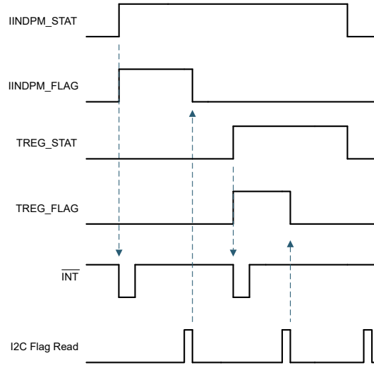
图 6-11. \overline{\text{INT}} 生成行为示例
