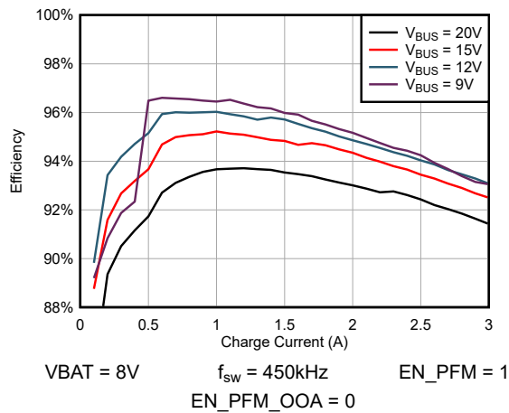
图 5-1. 2 节 充电效率与充电电流间的关系
