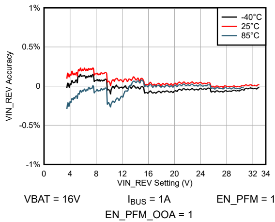
图 5-15. VIN_REV 精度
