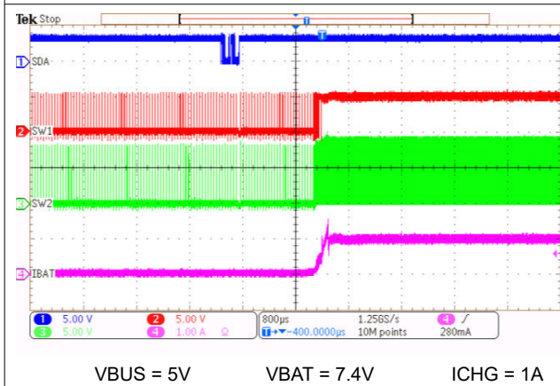
图 8-4. 通过 I 2 C 启用充电
