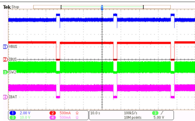
图 8-15. 没有 OOA 的正向升压模式 PFM
