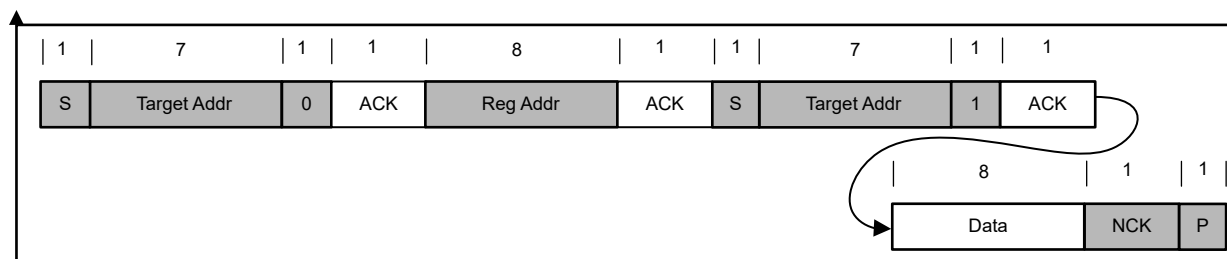
图 6-17. 单次读取
