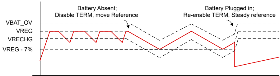
图 6-2. 电池检测
