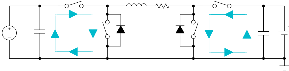
图 8-23. 转换器高频电流路径
