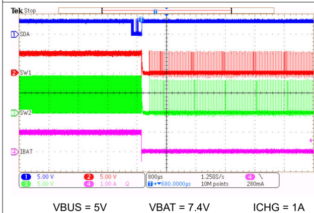
图 8-6. 通过 I 2 C 禁用充电
