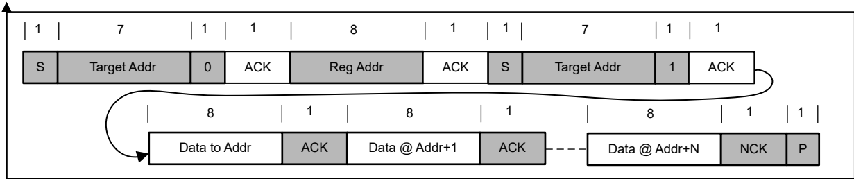
图 6-19. 多重读取
