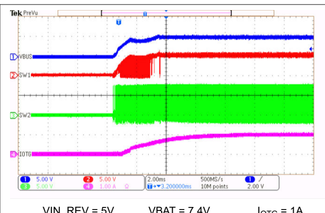
图 8-21. 在 1A OTG 负载下启用反向模式
