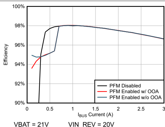
图 5-10. 不同 PWM/PFM/OOA 模式下 5 节串联电池 OTG 效率与充电电流间的关系
