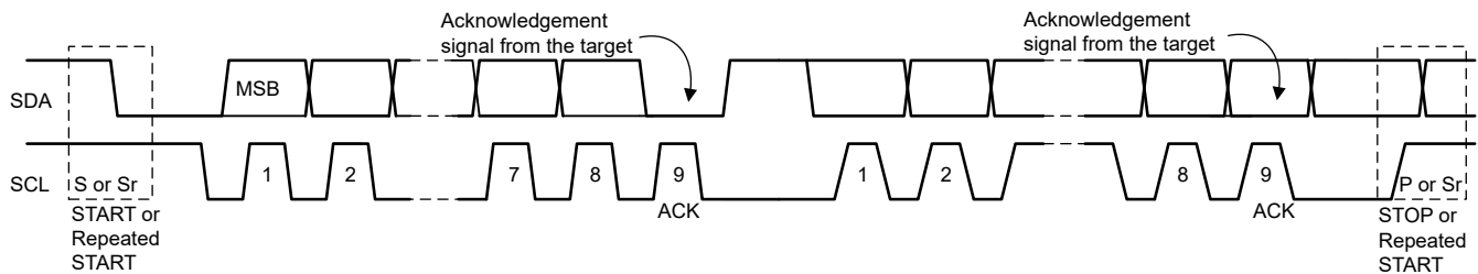
图 6-14. I 2 C 总线上的数据传输
