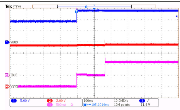
图 8-17. 低 VIN 下的 MPPT 调节
