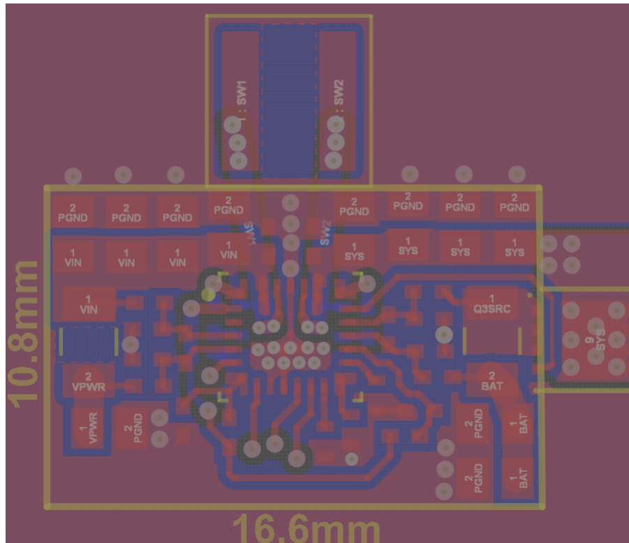
图 8-24. 2 层 PCB 布局示例的顶层 — 红色表示接地
