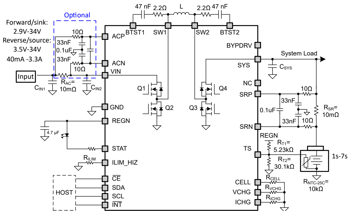
图 8-1. BQ25692-Q1 典型应用图
