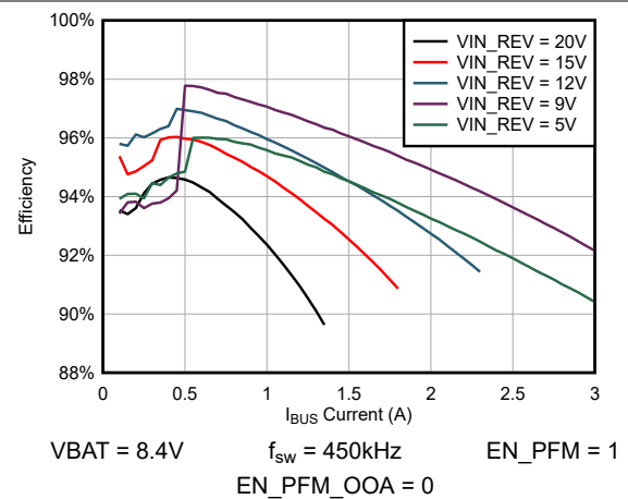
图 5-4. 2 节 电池 OTG 效率与 OTG 电流间的关系
