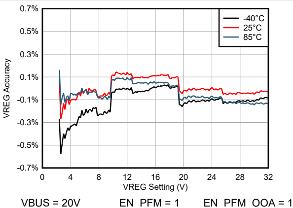
图 5-11. 充电电压精度
