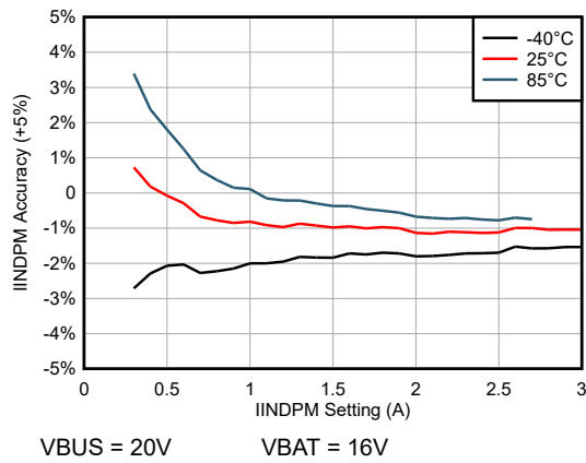
图 5-13. IINDPM 精度
