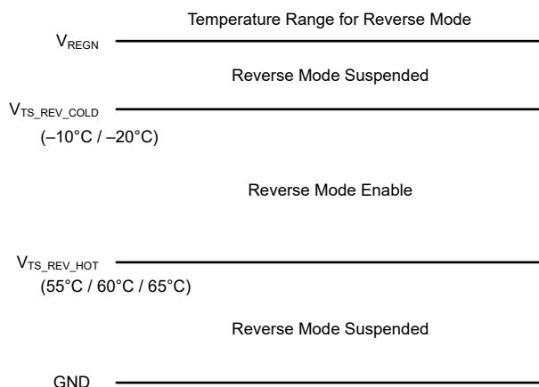
图 6-6. 反向模式下的 TS 引脚热敏电阻检测阈值
