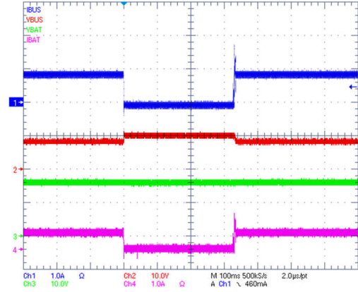
图 9-10. MPPT Operation Zoom
