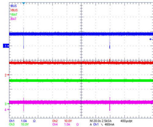
图 9-9. MPPT Operation
