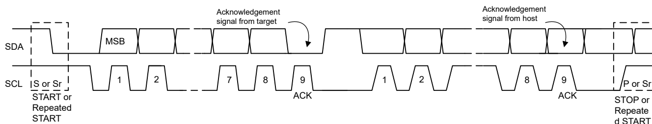
图 8-11. I 2 C 总线上的数据传输
