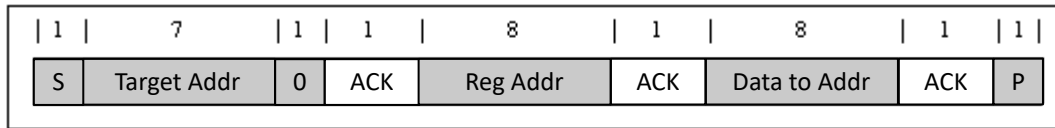
图 8-13. 单独写入
