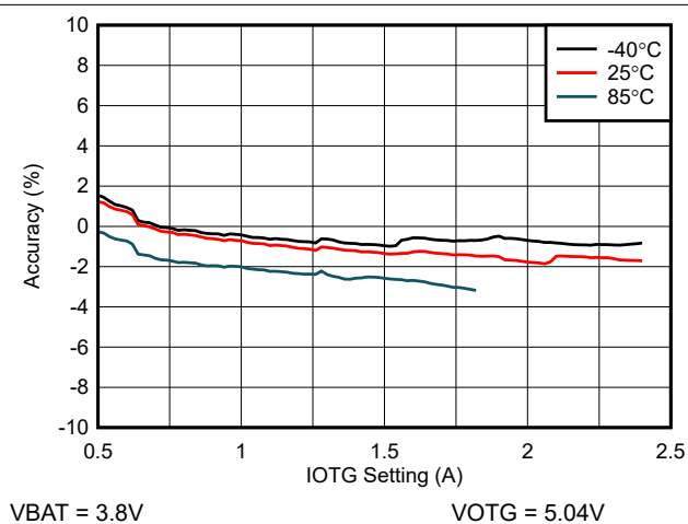
图 7-9. 升压电流调节精度与 IOTG 设置间的关系
