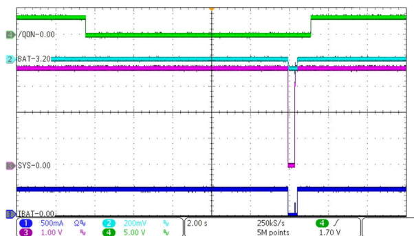
图 9-6. 充电禁用
