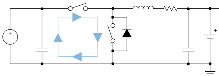
图 11-1. 高频电流路径
