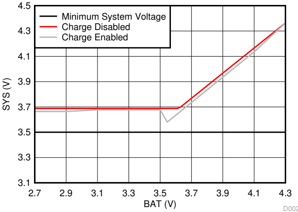
图 8-1. 系统电压与电池电压间的关系
