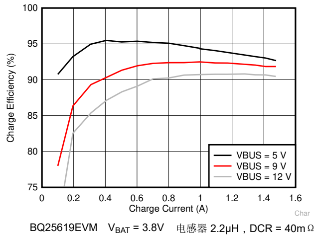
图 7-1. 充电效率
