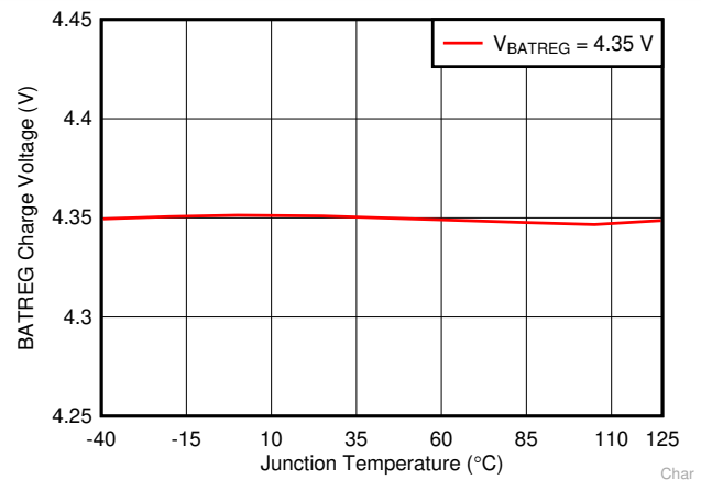
图 7-4. 电池充电电压与结温间的关系
