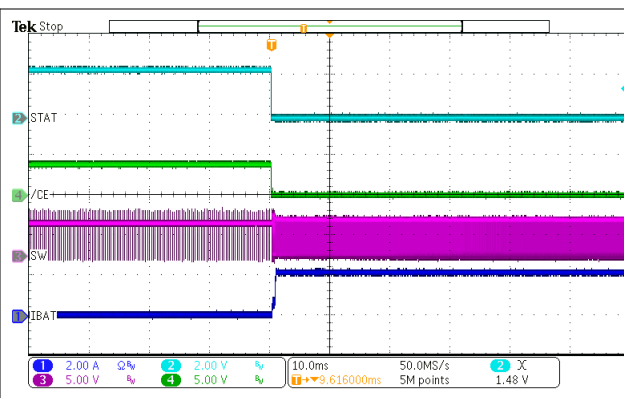
图 10-9. Charge Enable
