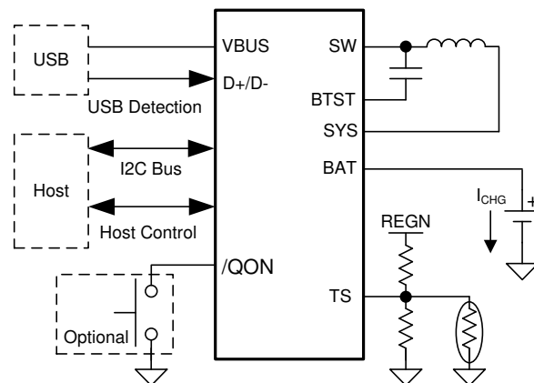
简化版应用
