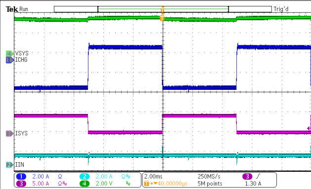
图 10-15. System Load Transient
