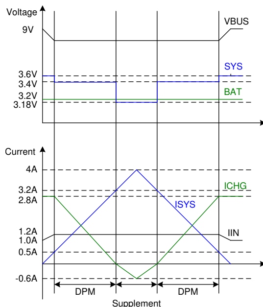
图 9-8. DPM Response
