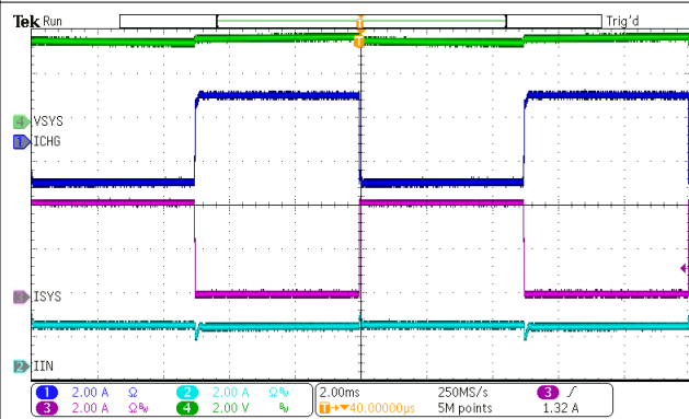
图 10-17. System Load Transient
