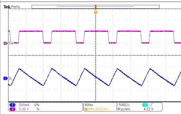
图 10-11. OTG Switching
