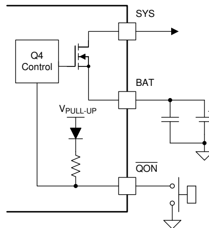
图 9-11. \overline{QON} Circuit
