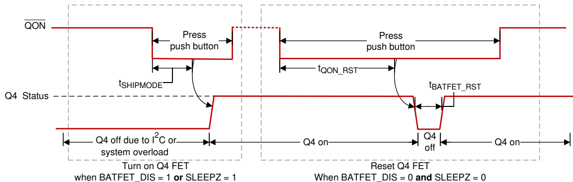
图 9-10. \overline{QON} Timing
