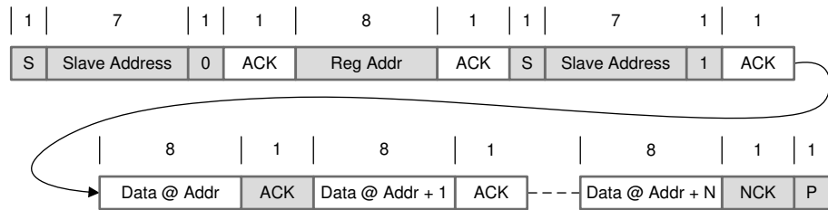
图 9-19. Multi-Read
