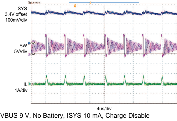
图 45. PFM Switching Waveform
