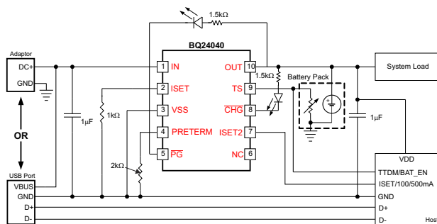
简化原理图
