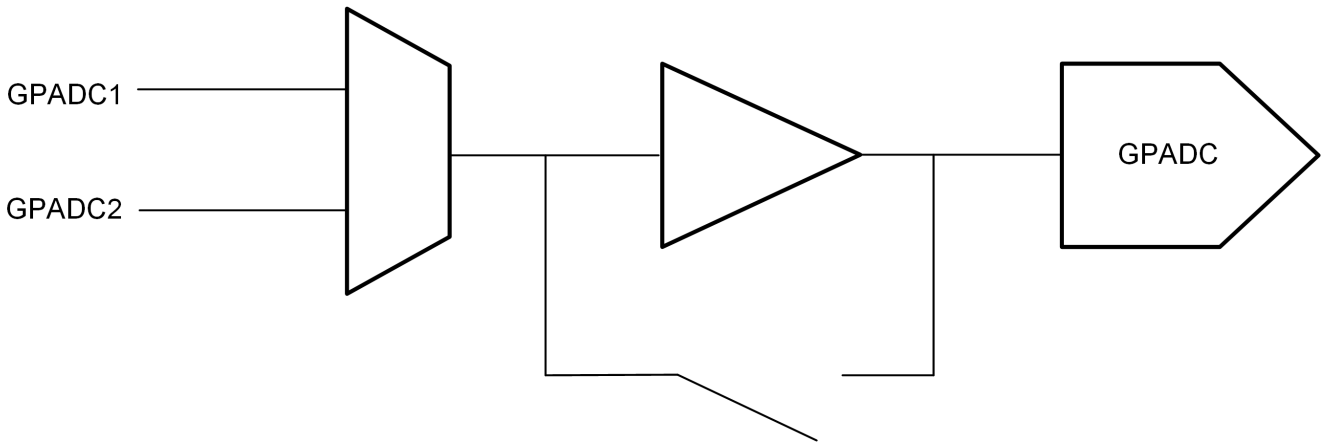
图 8-7. GPADC 路径
