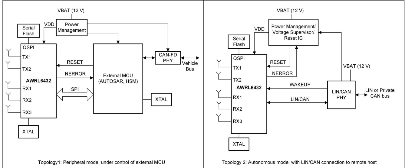
图 7-1. 系统拓扑
