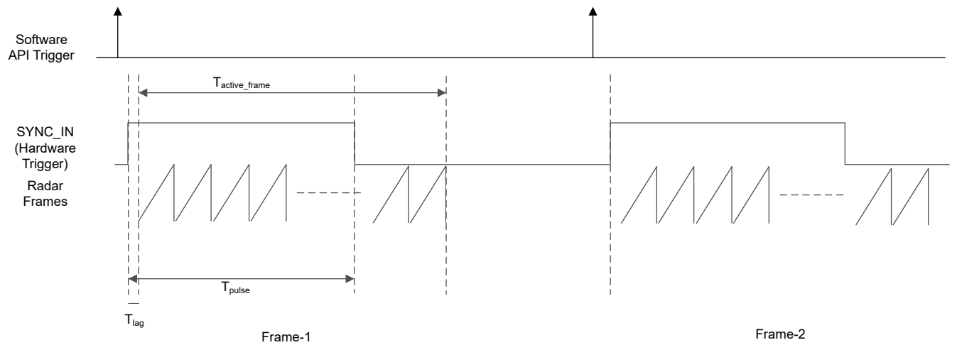
图 7-9. SYNC IN 硬件触发器
