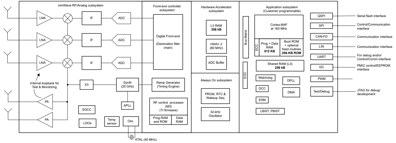
图 4-1. 功能方框图
