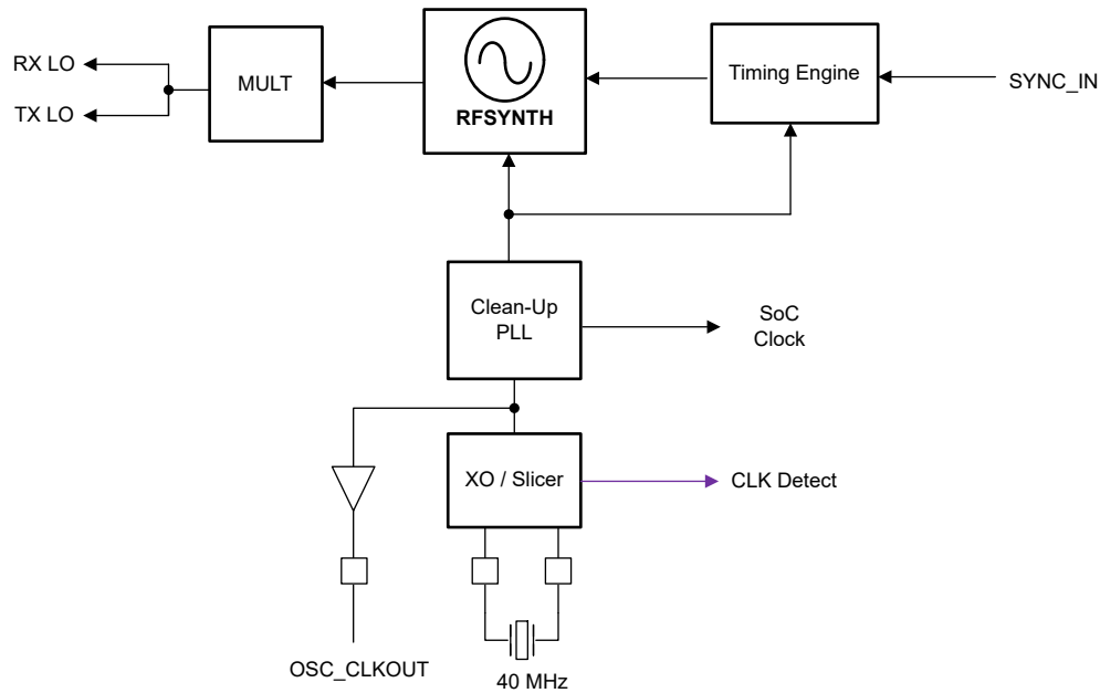
图 8-2. 时钟子系统
