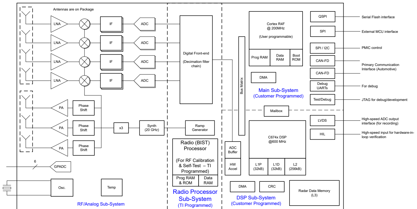
图 8-1. 功能方框图
