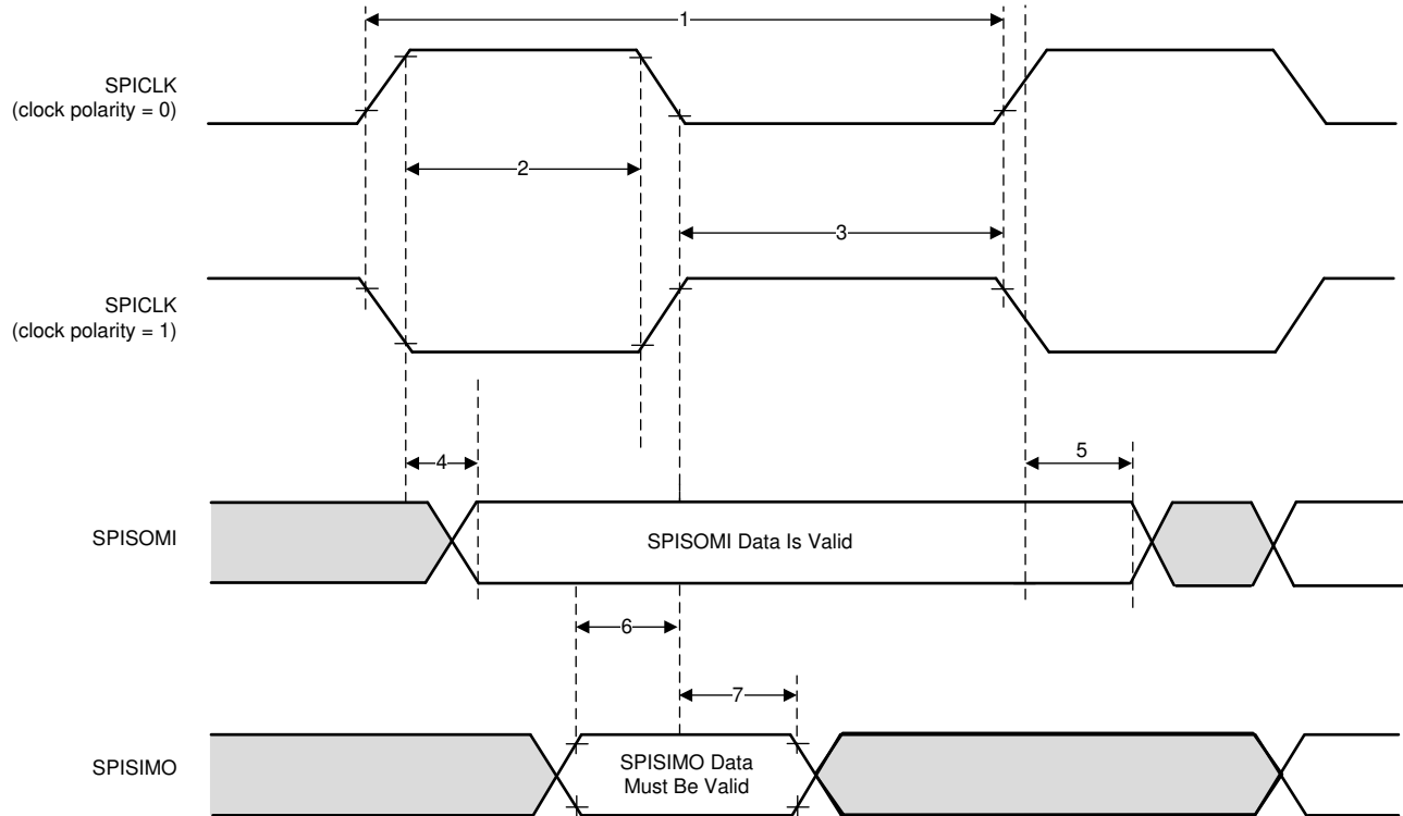
图 7-11. SPI 外设模式外部时序 (时钟相位 = 0)
