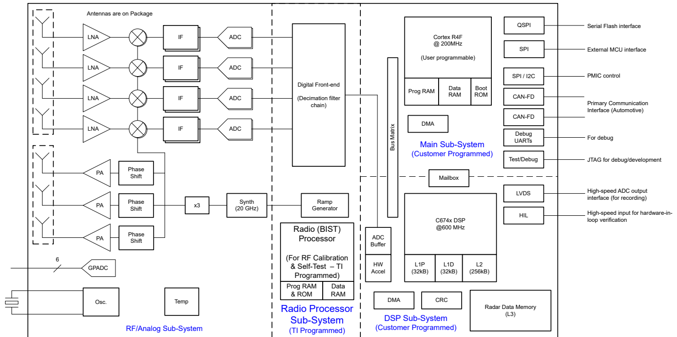
图 4-1. 功能方框图
