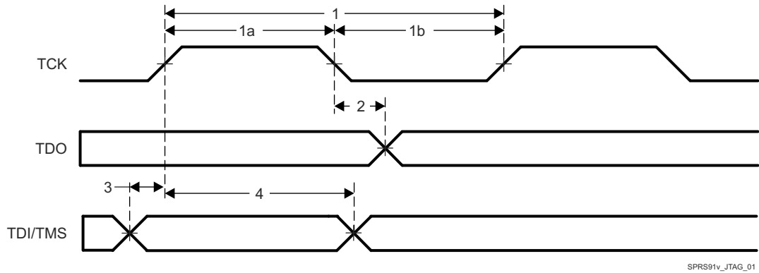
图 7-25. JTAG 时序
