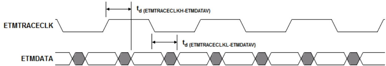
图 7-27. ETMDATA 时序
