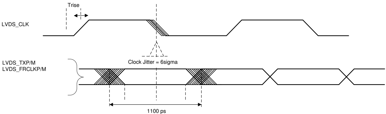
图 7-22. 计时参数
