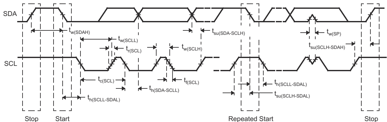
图 7-23. I2C 时序图
