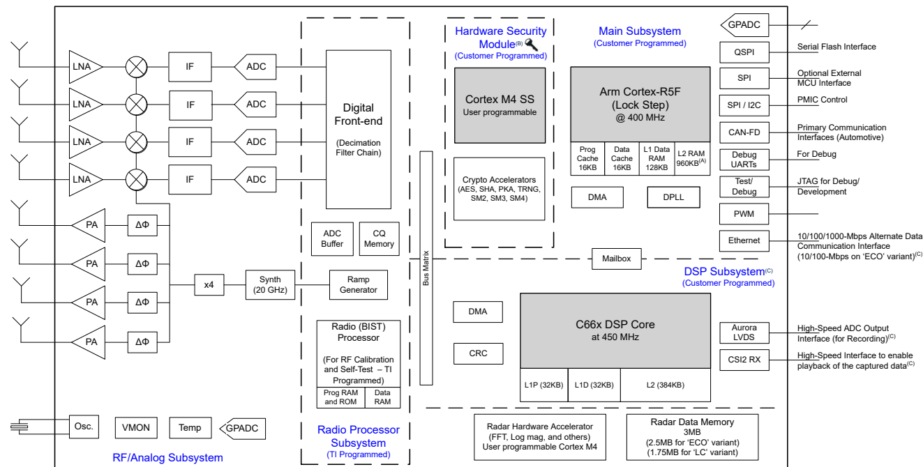
图 3-1. 功能方框图
