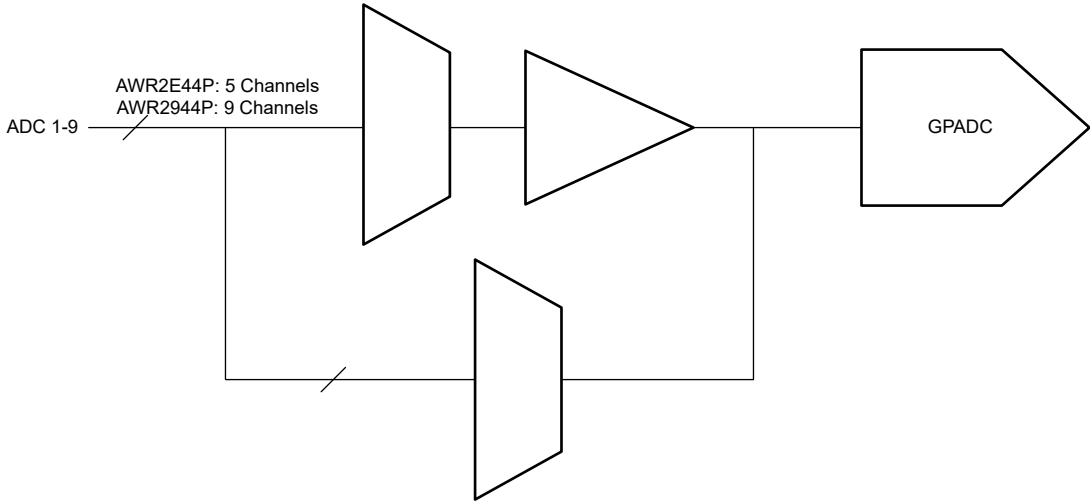
图 8-6. GPADC 路径
