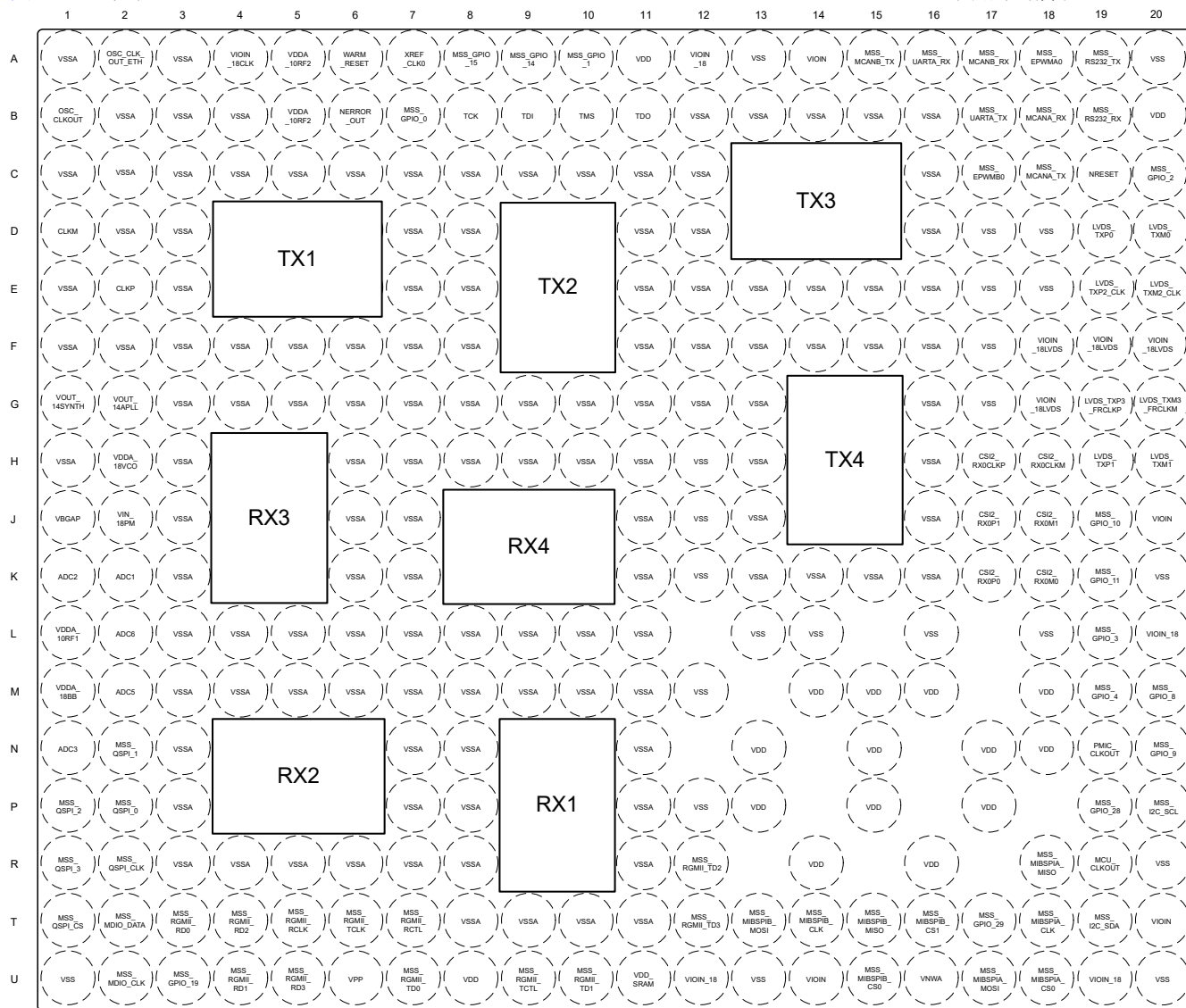
图 6-2. 引脚图 - AWR2E44P/AWR2E44-ECO/AWR2E44LC
