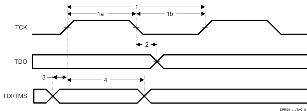
图 8-17. JTAG Timing
