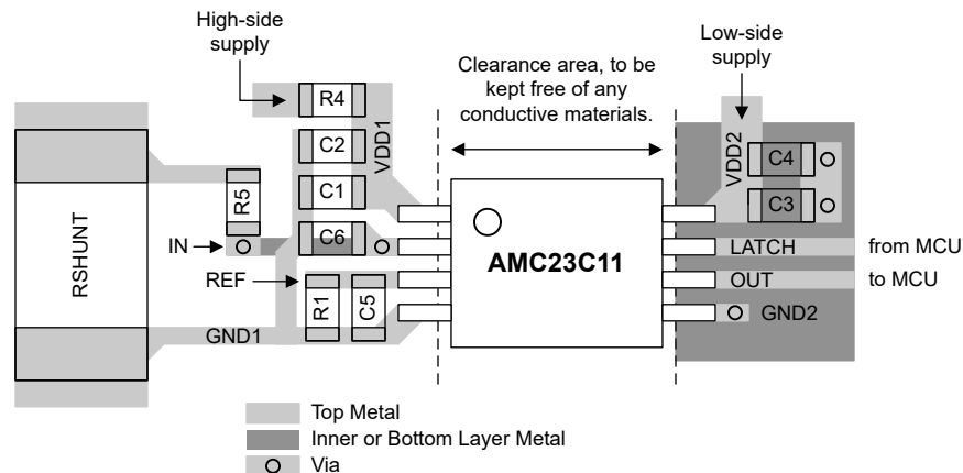
图 7-5. AMC23C11 的建议布局
