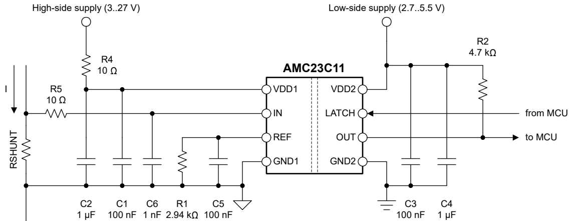
图 7-4. AMC23C11 去耦
