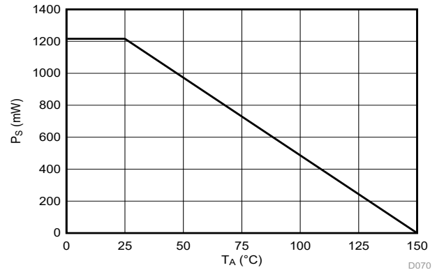
图 5-4. 安全限制功率的热降额曲线 (符合 VDE)
