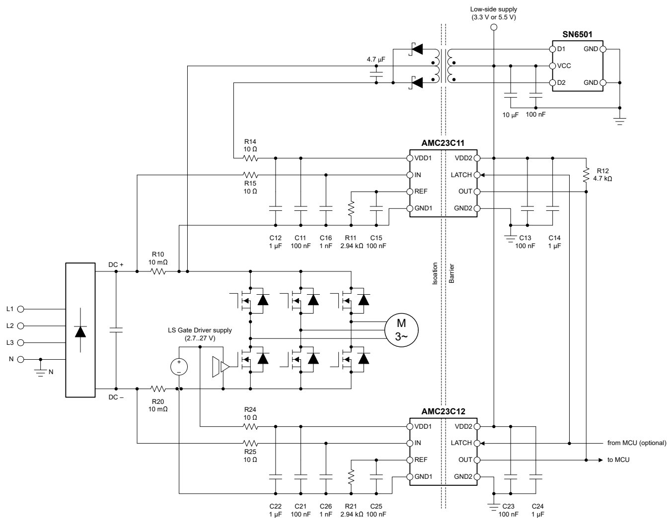
图 7-1. 使用 AMC23C11 进行 DC+ 过流检测
