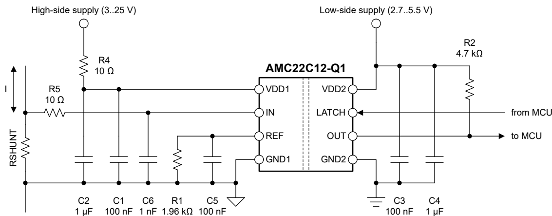
图 7-6. AMC22C12-Q1 去耦
