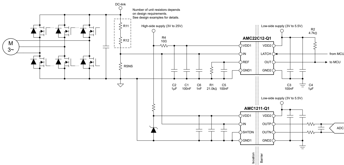
图 7-2. 使用 AMC22C12-Q1 进行过压检测
