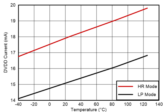
图 6-17. DVDD 电流与温度间的关系
