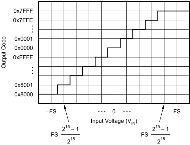
图 8-23. 代码转换图
