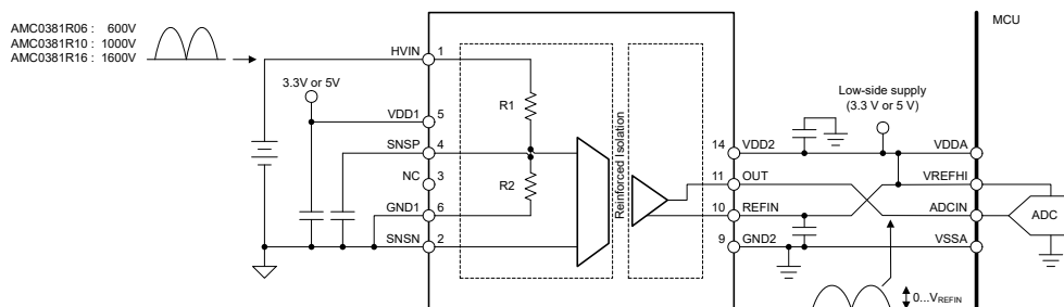
典型应用 (DFX 封装)
