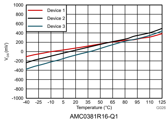
图 6-16. 输入失调电压与温度间的关系
