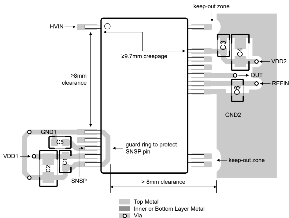
图 8-6. AMC0381R-Q1 ( DFX 封装 ) 的建议布局
