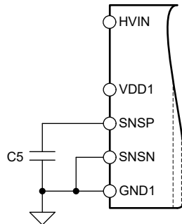
图 8-2. 输入滤波器
