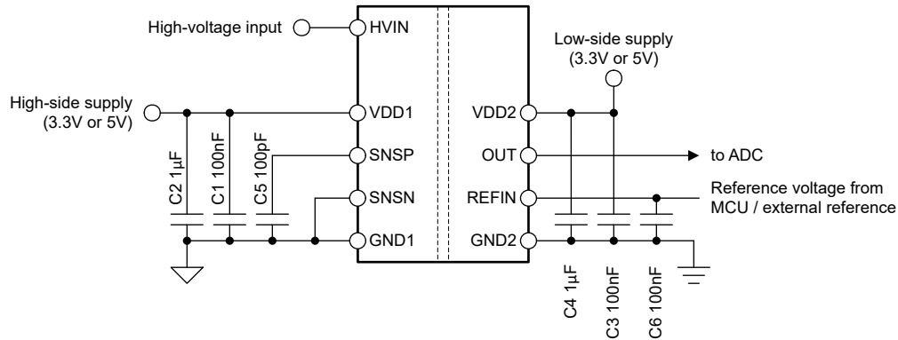
图 8-5. AMC0381R-Q1 去耦
