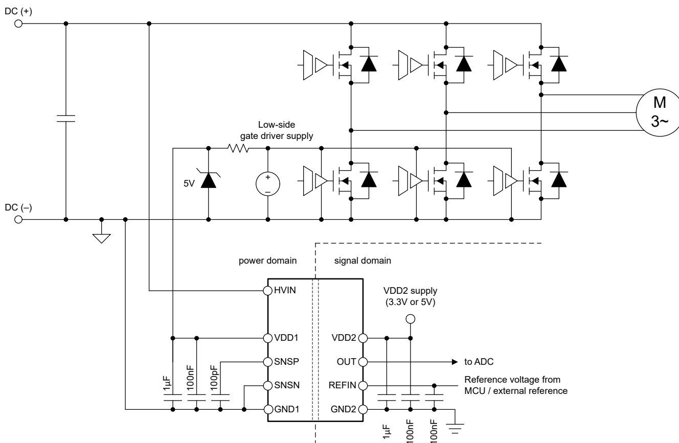
图 8-1. 在典型应用中使用 AMC0381R-Q1
