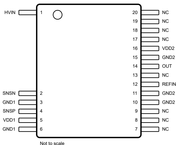
图 5-2. DFJ 封装，20 引脚 SOIC ( 顶视图 )
