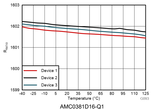
图 6-10. 分压器分压比与温度间的关系
