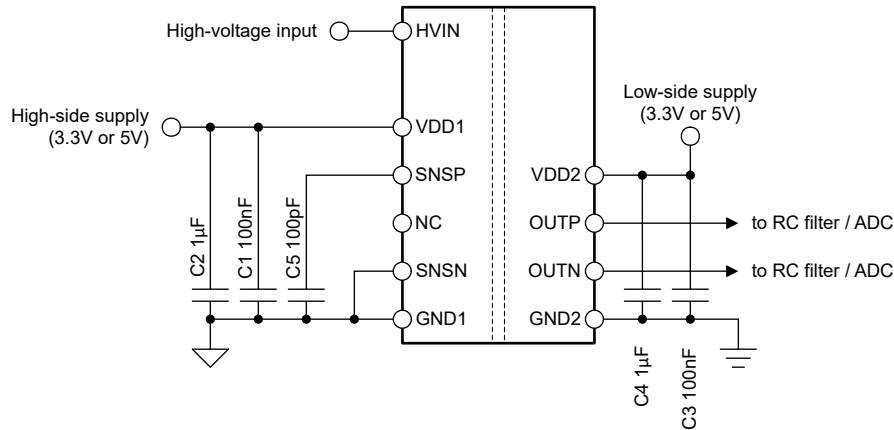
图 8-5. AMC0381D-Q1 去耦
