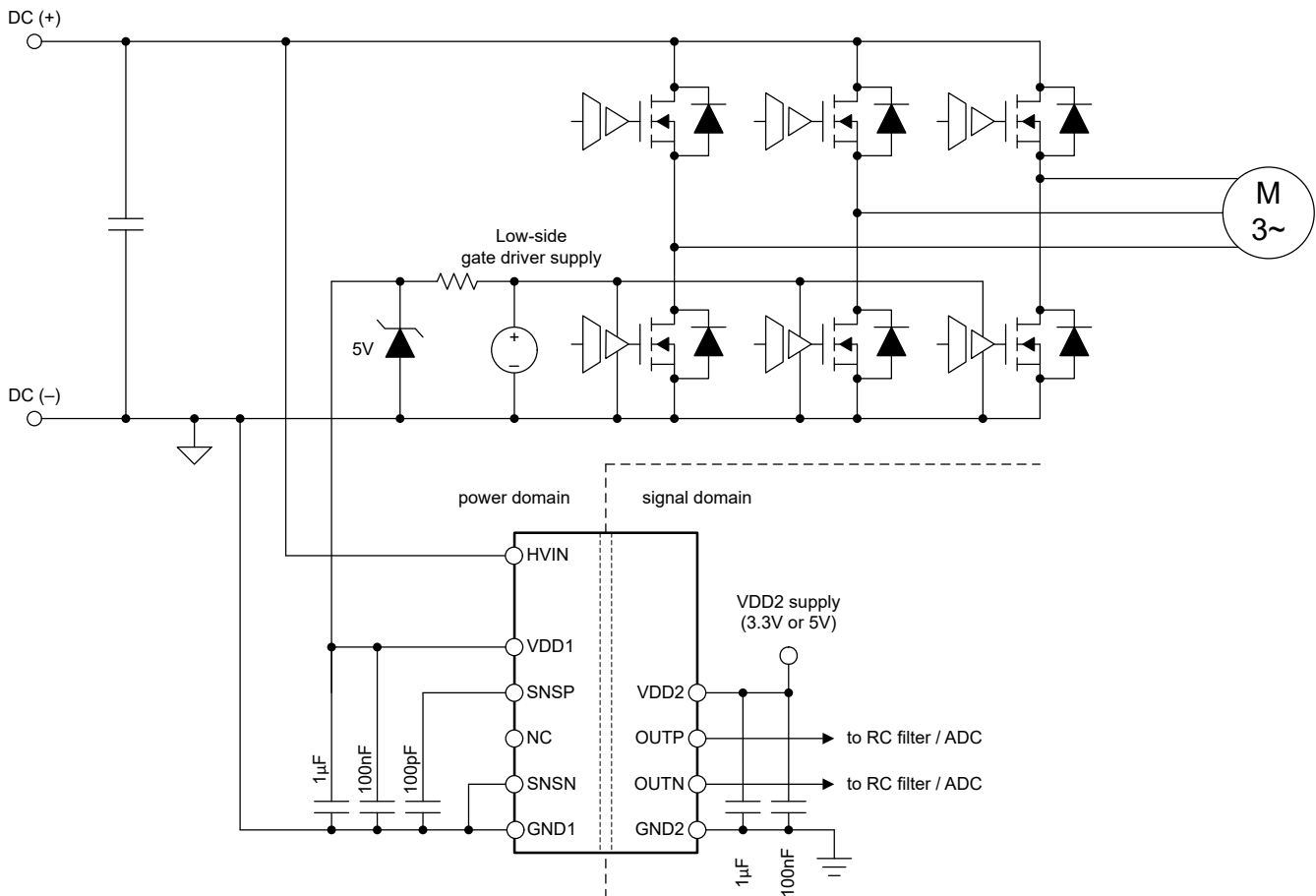
图 8-1. 在典型应用中使用 AMC0381D-Q1
