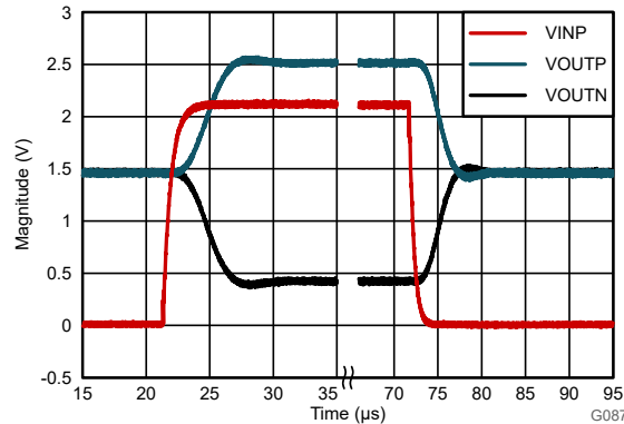
图 8-4. AMC0381D-Q1 的阶跃响应
