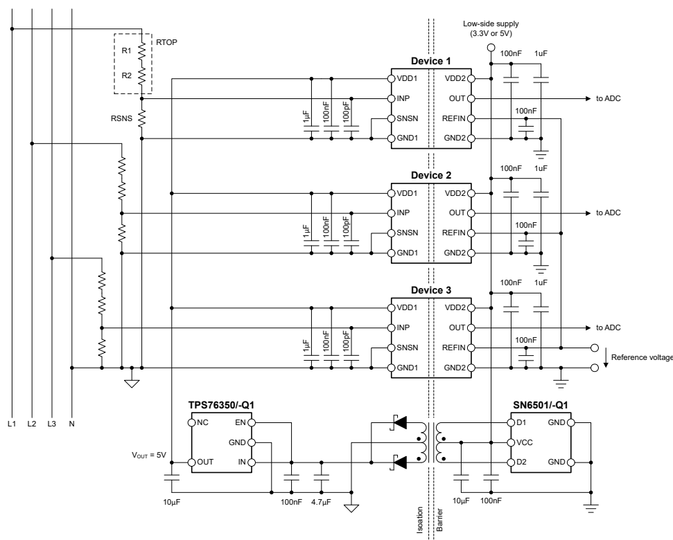
图 8-1. 在典型应用中使用 AMC0x30S
