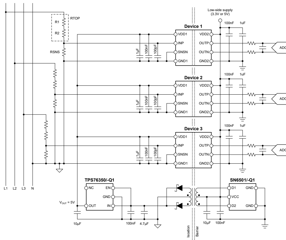
图 8-1. 在典型应用中使用 AMC0x30D-Q1
