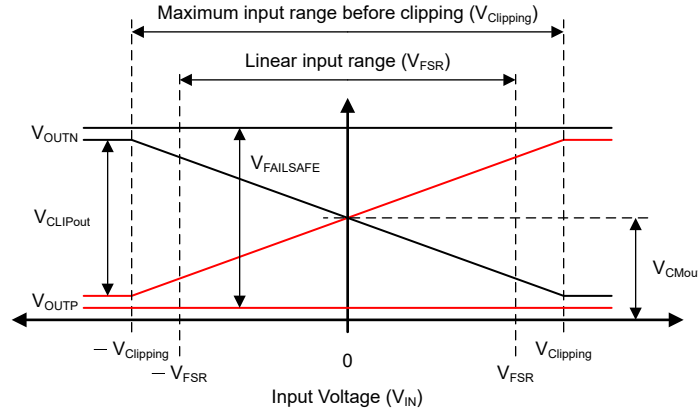
图 7-2. AMC0x30D-Q1 的输入到输出传递曲线
