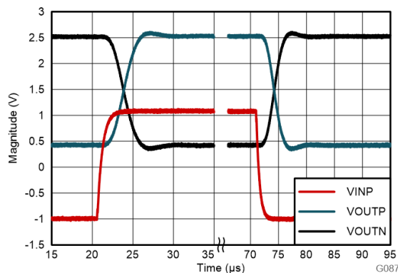
图 8-4. AMC0x30D-Q1 的阶跃响应
