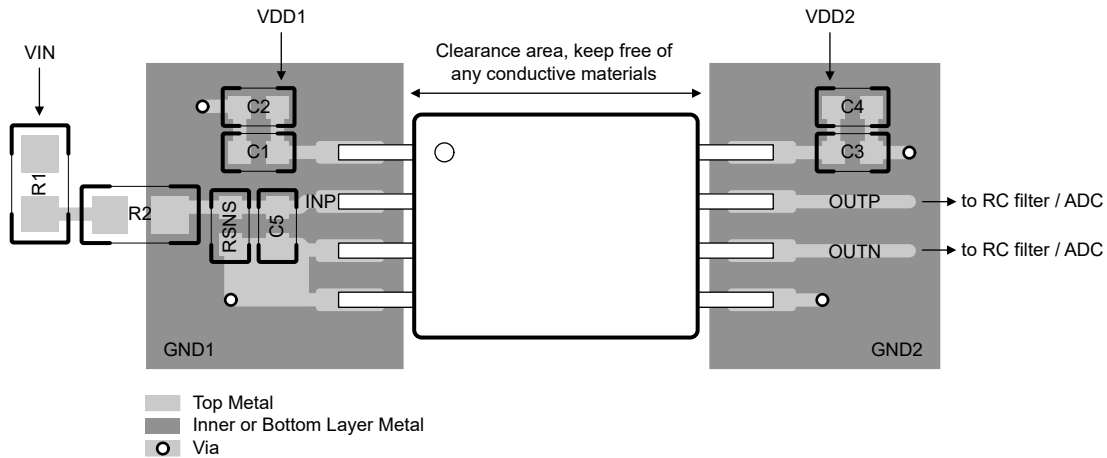
图 8-6. AMC0x30D-Q1 的建议布局
