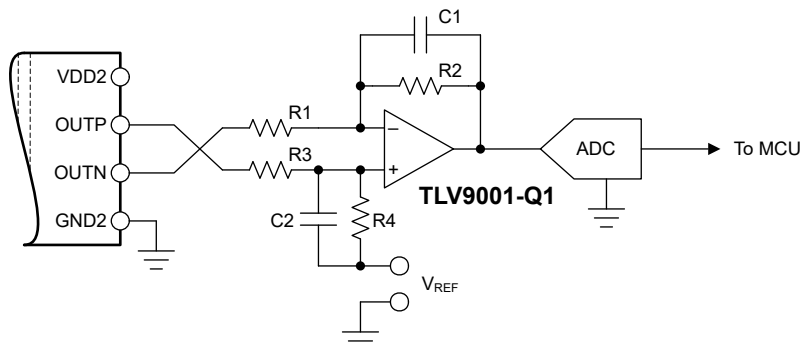
图 8-3. 将 AMC0x30D-Q1 输出连接到单端输入 ADC
