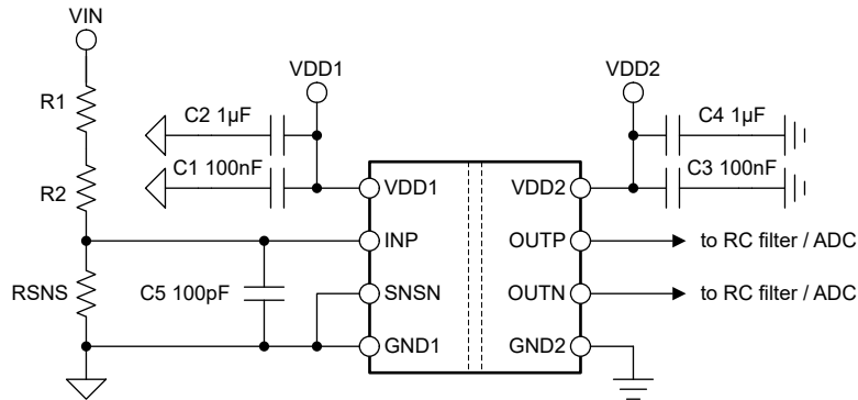
图 8-5. AMC0x30D-Q1 去耦
