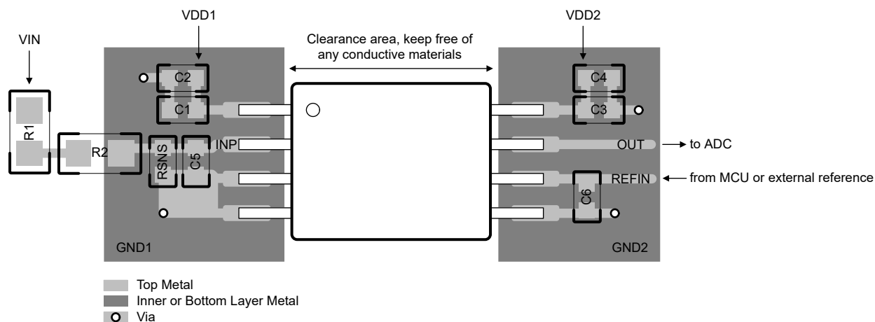
图 8-6. AMC0x11R-Q1 的建议布局
