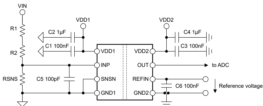
图 8-5. AMC0x11R-Q1 去耦
