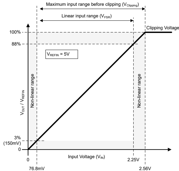
图 7-2. AMC0x11R-Q1 的输入到输出传送曲线
