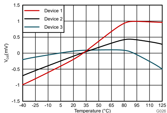
图 6-7. 输入失调电压与温度间的关系
