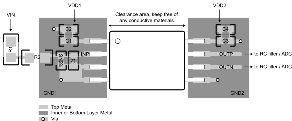
图 8-6. AMC0x11D-Q1 的建议布局
