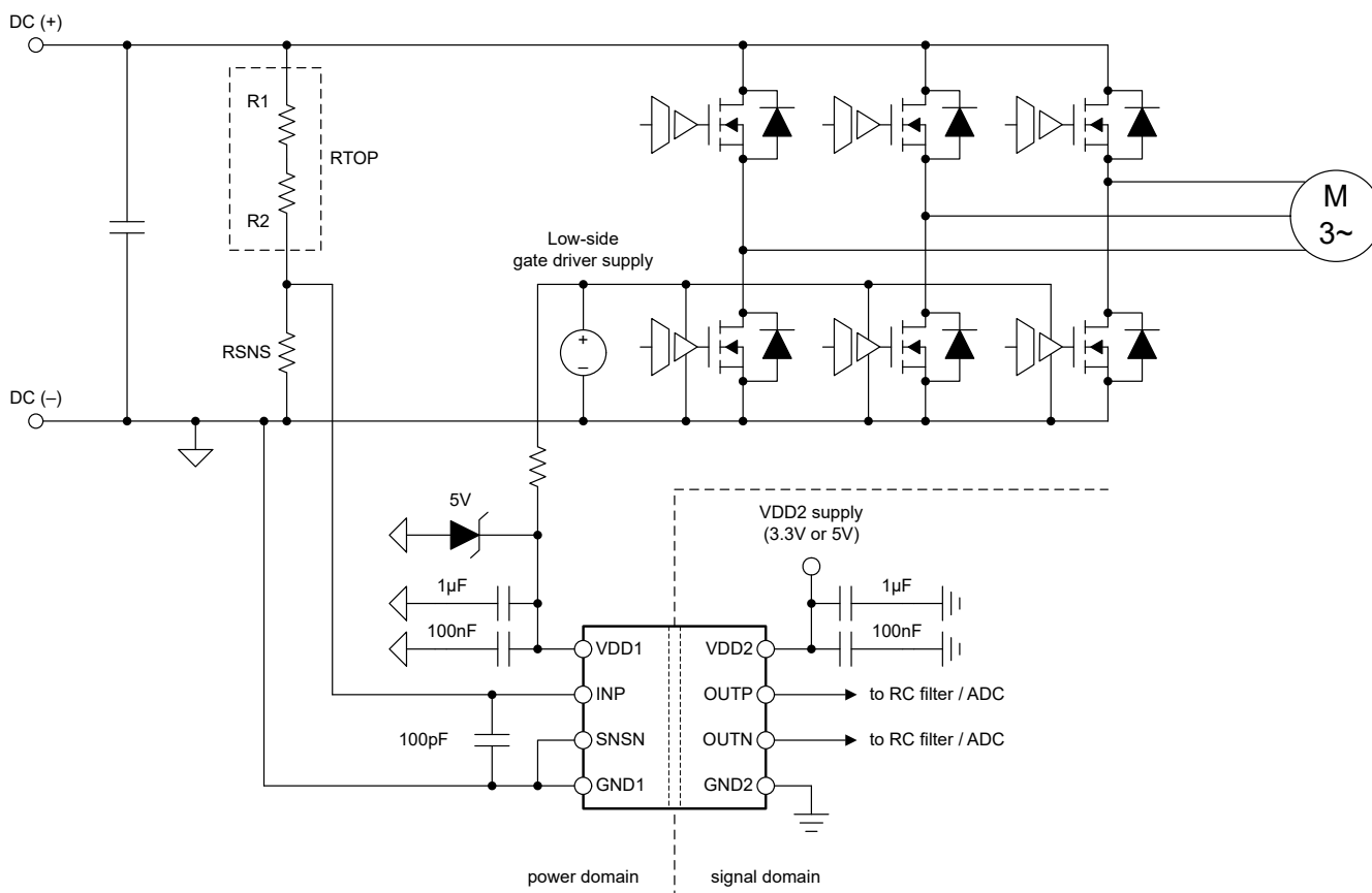
图 8-1. 在典型应用中使用 AMC0x11D-Q1
