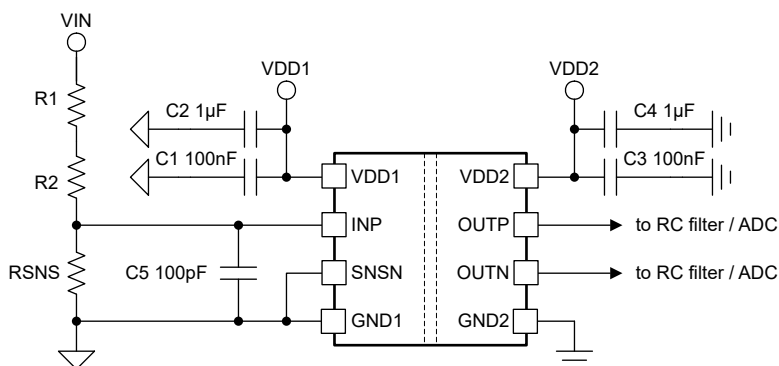
图 8-5. AMC0x11D-Q1 去耦
