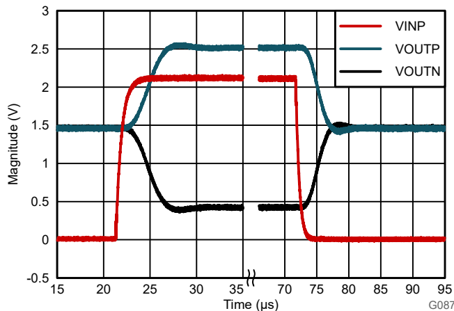
图 8-4. AMC0x11D-Q1 的阶跃响应
