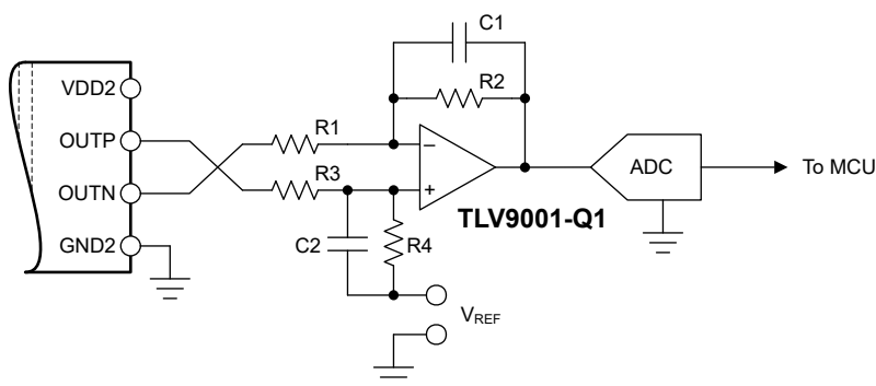
图 8-3. 将 AMC0x11D-Q1 输出连接到单端输入 ADC
